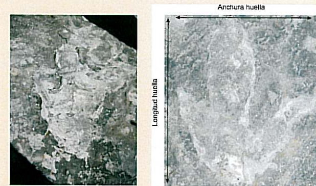
En el estrato que contiene a las huellas tridáctilas es posible observar fragmentos de invertebrados marinos.
