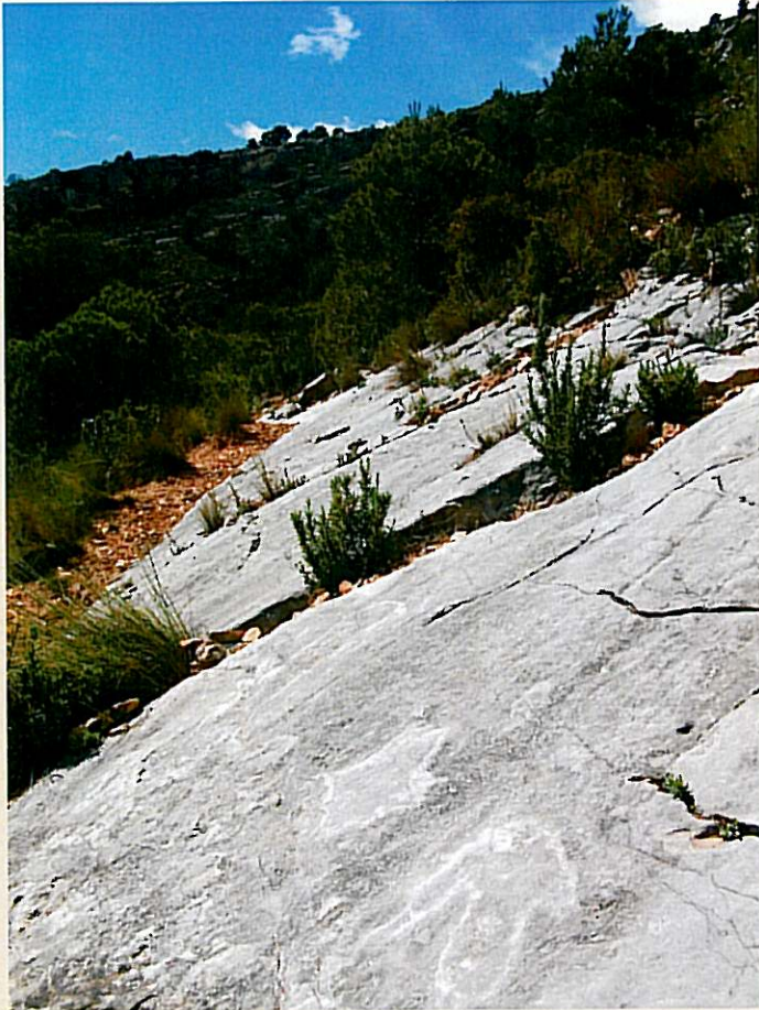
Estrato rocoso con las icnitas en Abenfigo.
