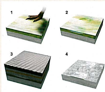
Esquema de formación de las icnitas.
