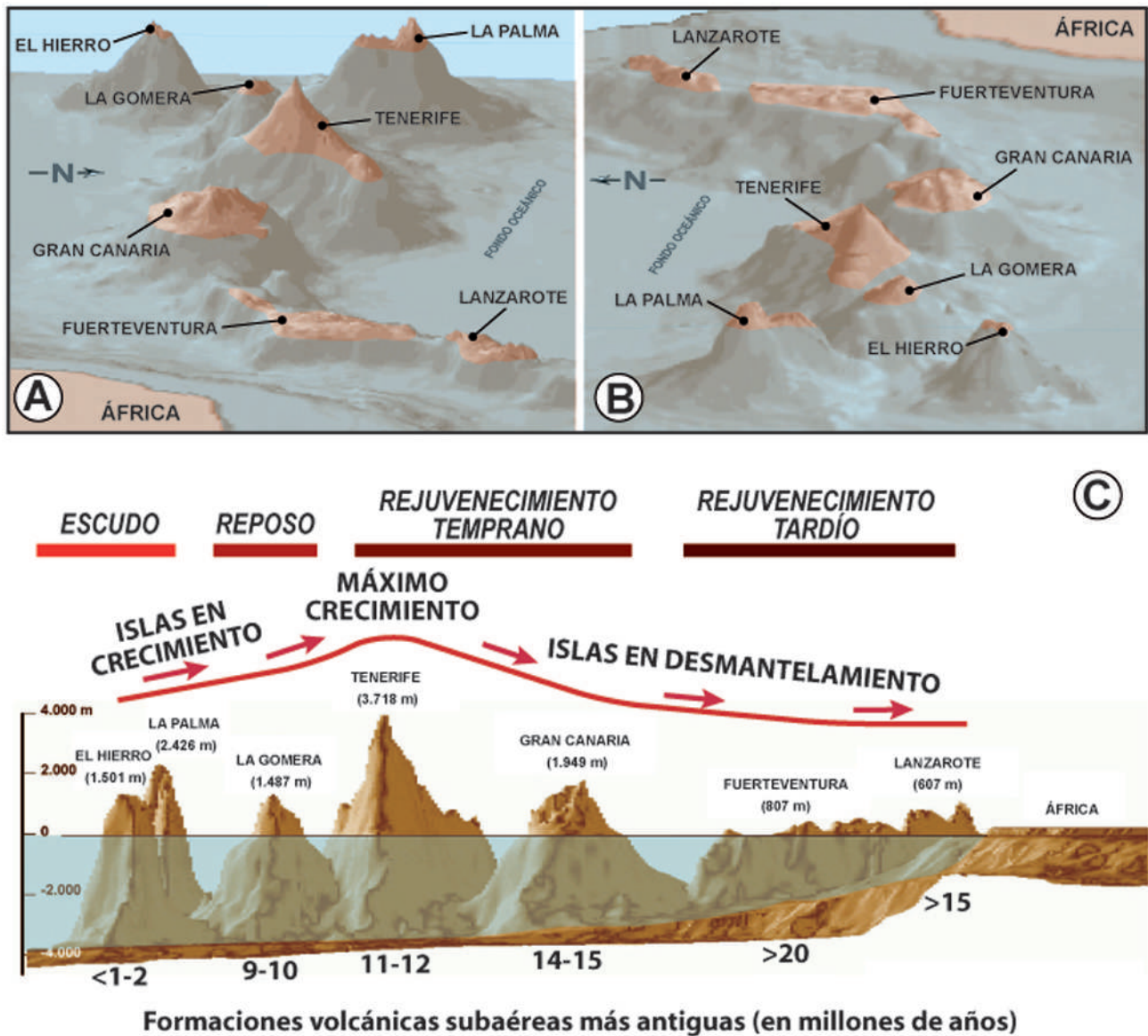
Figura 1. A) Simulación por ordenador del área de las Islas Canarias a océano vacío vista de Este a Oeste. B) Ídem. de Oeste a Este. C) Perfil del archipiélago mostrando la edad de nacimiento, etapa de evolución y máximas alturas de las diferentes islas.
