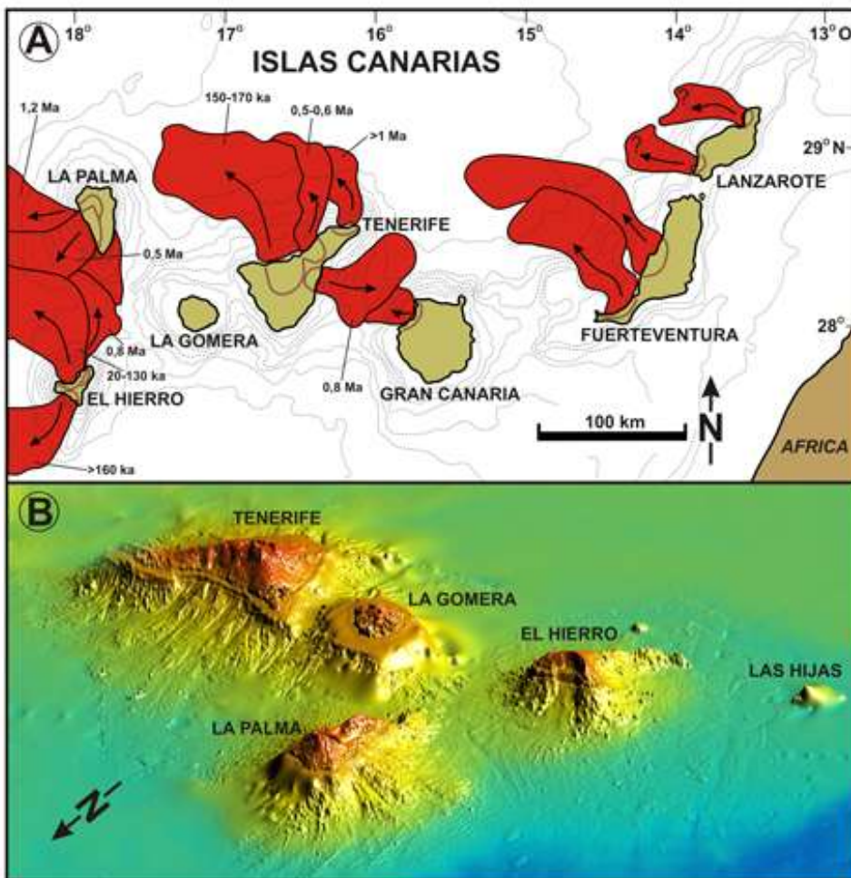
Figura 2. A) Deslizamientos laterales gigantes en las Islas Canarias (los números indican sus edades estimadas; Ma, en millones de años; ka, en miles de años) y conexión con calderas de colapso en tierra. B) Imagen de sonar de las islas occidentales, vistas de NE a SO, en la que se puede observar el escaso desarrollo de las plataformas insulares en las islas de Tenerife, La Palma y El Hierro, mientras que en La Gomera son muy anchas. Asimismo, destacan los volcanes submarinos bautizados como "Las Hijas" que en un futuro geológico pueden llegar a constituir nuevas islas.
