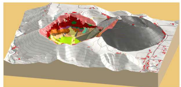
6. Visión oblicua actual de la Caldera y el Pico de Bandama desde el Este
