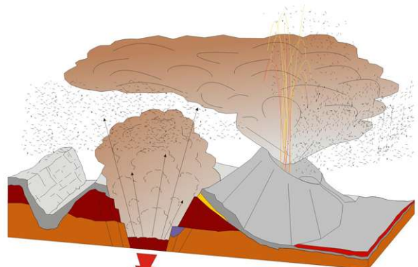
5. Debilitado por las fuertes explosiones el relieve colapsa hundiéndose. Se forma la Caldera de Bandama. La actividad piroclástica del Pico de Bandama terminará poco más tarde
