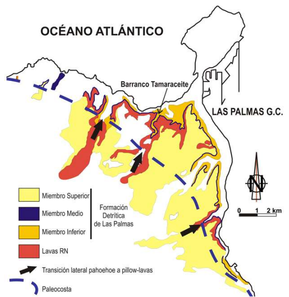
Figura 4. Esquema geológico del NE de Gran Canaria. Obsérvese la posición de la línea de costa hace unos 4 m.a., donde el mar llegaba a estar unos 100 metros más alto que el actual. Las lavas del estratovolcán Roque Nublo llegaron a formar una especie de "delta" que ganó al mar una superficie de unos 25 km 2 . El nacimiento de La Isleta hace 1 m.a., la formación de un tómbolo de arena que la terminaría uniendo al resto de la isla (donde hoy se asienta gran parte de la ciudad de Las Palmas de Gran Canaria) y las últimas oscilaciones del nivel del mar han dado lugar a la morfología de la línea de costa actual.
