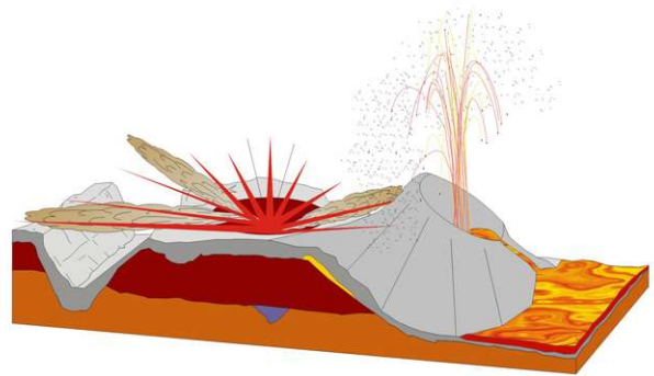
4. Continúan las erupciones explosivas en el cono S ensanchando el cráter del edificio. Desde la base del cráter del cono N surge una potente colada de lava que se canaliza a través del Valle de los Hoyos
