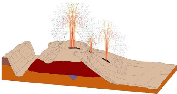
1. Relieve anterior a la erupción, en el que una fisura eruptiva N-S expulsa surtidores de cenizas
