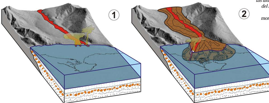
Figura 5. Secuencia de relleno de la paleobahía somera que existía en los alrededores de la ciudad de las Palmas hace unos 4 m.a. Se indica el contorno actual de la costa en esta zona para comparar.
