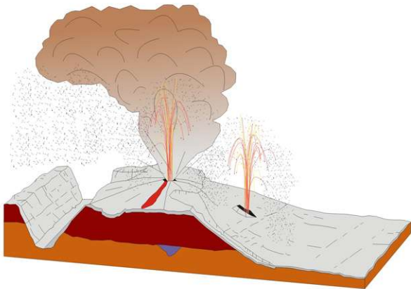
2. La actividad se concentra en los extremos N y S de la fisura en donde crecen desigualmente dos conos volcánicos (futura Caldera en el extremo S y futuro Pico en el extremo N). Desde el Sur se emite una colada de lavas. Las cenizas cubren el entorno
