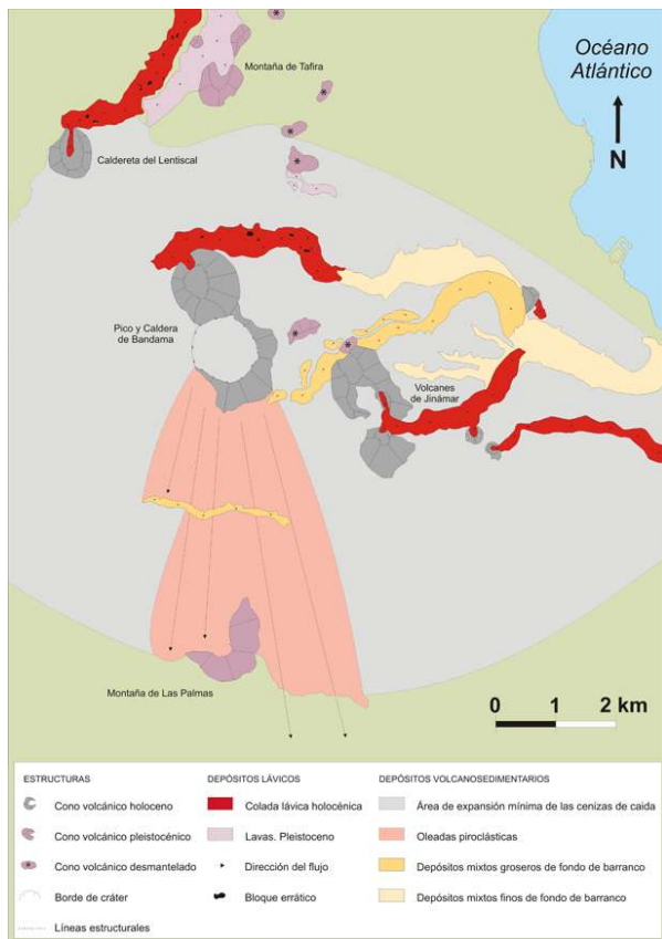
Figura 6. Mapa geológico de los volcanes Holocenos del NE de Gran Canaria. Destacan el Pico y La Caldera de Bandama como los volcanes más importantes y recientes.
