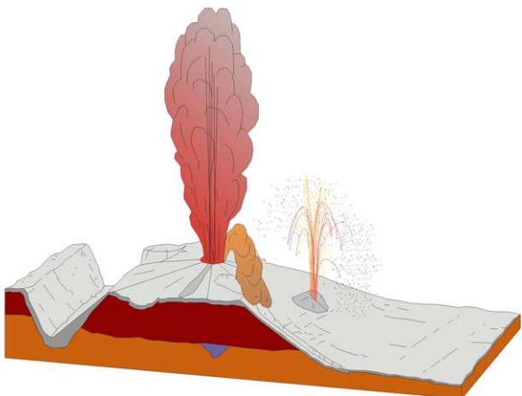
3. Contacto de la chimenea S con agua subterránea e inicio de erupciones muy explosivas freatomagmáticas
