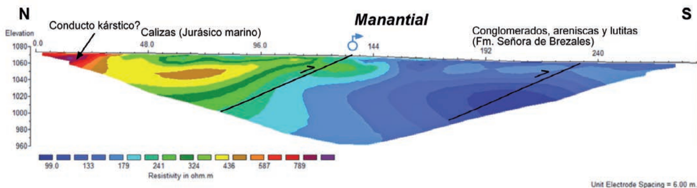
Fig. 2.- Tomografía eléctrica realizada en las proximidades del manantial. Nótese que la escala horizontal es mayor que la vertical, lo que hace que las fallas parezcan más tendidas de lo que son. La posición de la tomografía se indica en la figura 1. Ver figura en color en la web.
