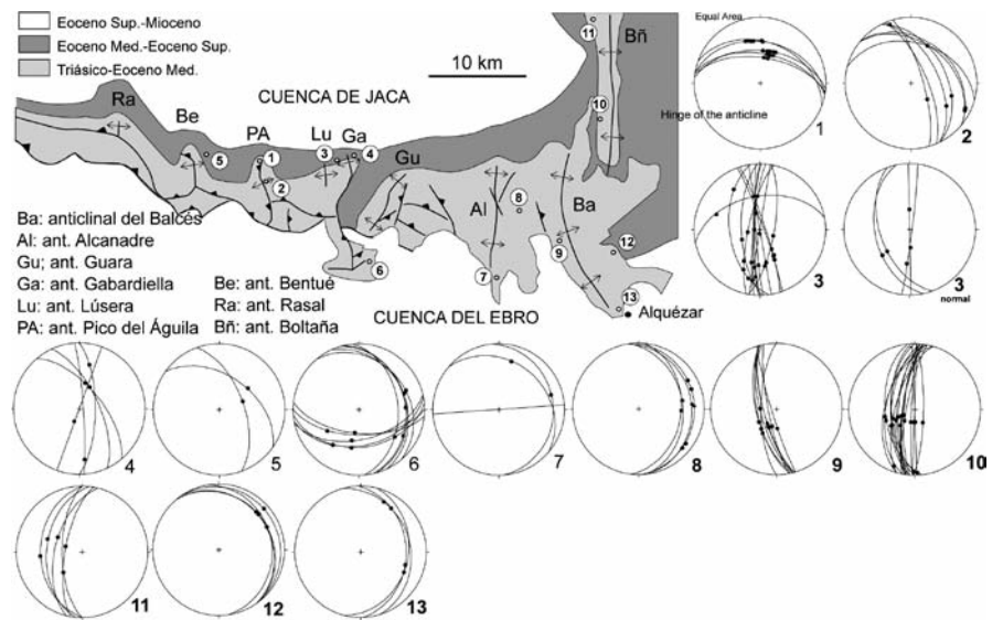
Fig. 3.- Indicadores cinemáticos (puntos negros) tomados sobre plano de estratificación (ciclográficas). Las estereográficas representan el hemisferio inferior y son equiareales.
