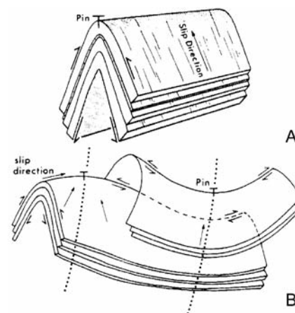
Fig. 1.- Mecanismo de flexural-slip en pliegues cilíndricos (A) y no cilíndricos (B). Modificado de Tanner (1989).
