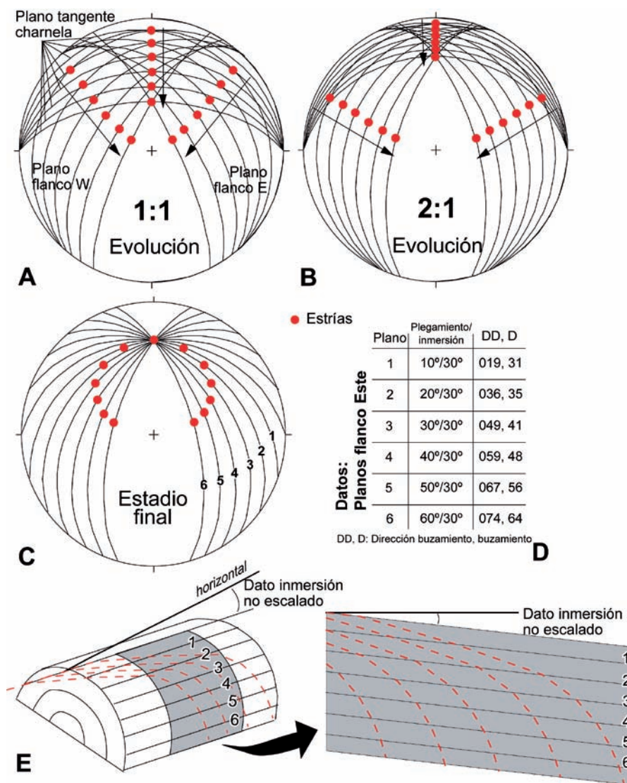
Fig. 5.-Modelo B. Plegamiento e inmersión simultáneos. Evolución cinemática de un plano tangente a la charnela y dos pertenecientes a los flancos E y W de un pliegue cilíndrico (A) con incrementos de 10° de plegamiento y 10° de inmersión en cada etapa y (B) con incrementos de 20° de plegamiento y 10° de inmersión en cada etapa. (C-E) Estadio final para planos con distinto buzamiento pertenecientes al mismo pliegue cilíndrico (datos referidos a plano de flanco E) con plegamiento e inmersión simultáneos 2:1.
