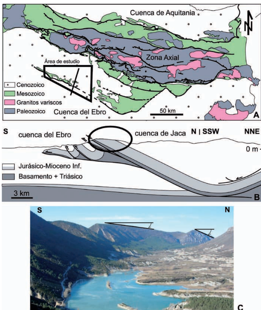
Fig. 2.- A) Localización del área de estudio en el Pirineo. B) Corte geológico esquemático mostrando como los pliegues N-S de las Sierras Exteriores Aragonesas se sitúan sobre una rampa de bloque inferior buzando al N de media 30° (modificado de Millán et al. , 2000). C) Anticlinal de Bentué desde el anticlinal Pico del Águila situado al E donde se observa su inmersión al N. Ver figura en color en la web.
