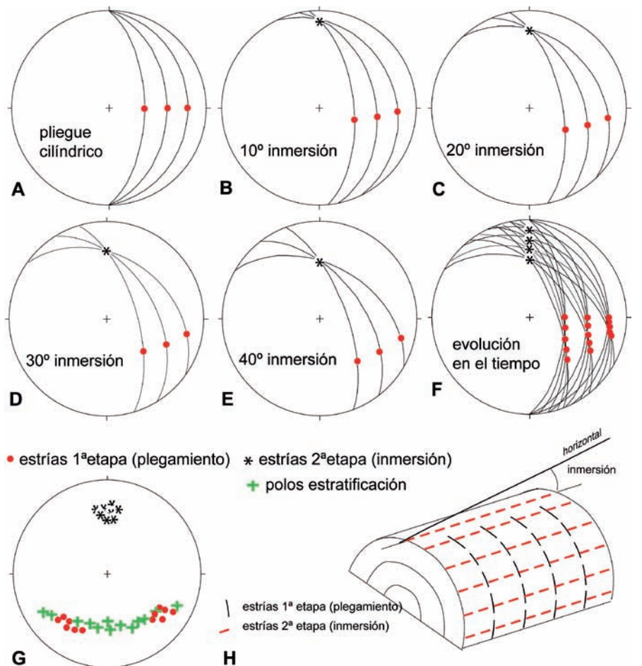
Fig. 4.- Modelo A. Plegamiento e inmersión no simultáneos. Evolución cinemática del flanco oriental de un pliegue cilíndrico horizontal con inmersión posterior (A-F). Ejemplo de la etapa final para ambos flancos (G). Ejemplo pliegue cilíndrico con las dos familias de estrías (H).
