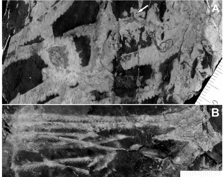
Fig. 3.- Graptolitos extensiformes del Ordovícico del Sinclinal de Rececende. A, región proximal de Expansograptus? sp. 1, con la sícula señalada con una flecha; debajo del ejemplar se aprecian fragmentos de otros estipes muy anchos ( Expansograptus? sp. 2); B, fragmentos distales de estipes de Expansograptus? sp. 1. Todos los ejemplares ilustrados se muestran orientados de igual manera frente a la lineación tectónica principal, que induce ensanchamiento perpendicular al eje de los estipes. Escala en mm.
