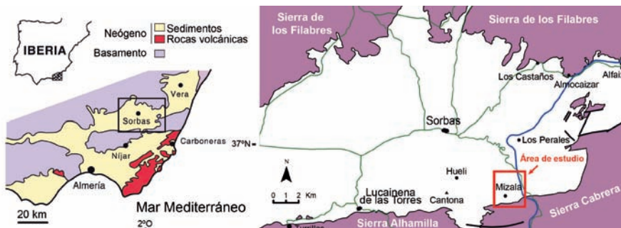
Fig. 1.- Localización de la Cuenca de Sorbas (izquierda) y del área estudiada (derecha). Ver figura en color en la Web.
