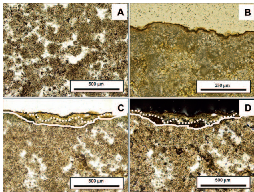
Fig. 3.-A-Imagen con nicoles paralelos de la dolomía microcristalina equigranular hipidiotópica que constituye el substrato de las muestras de pátinas tomadas en la iglesia del Salvador y del convento de Santo Domingo (Cifuentes, Guadalajara). B- Imagen con nicoles paralelos de la pátina de la fachada sureste del convento de Santo Domingo, en la que se observa la pátina como una fina capa de color anaranjado. C y D.- Imágenes con nicoles paralelos (C) y cruzados (D) de la pátina de la entrada de la fachada sur de la iglesia del Salvador; se distingue una capa anaranjada exterior y una capa isotrópica interior que se sitúa en contacto con el substrato. La línea continua señala el contacto entre pátina y substrato mientras que la línea de puntos marca el contacto entre las dos capas que constituyen la pátina.
