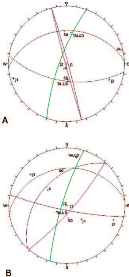
Fig. 2.- Diagramas de planos y polos de las estaciones geomecánicas 1 (A) y 2 (B).
