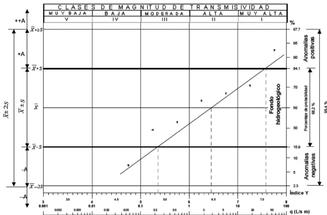
Fig. 3. Distribución de la transmisividad en carbonatos alpujárrides. Interpretación basada en el gráfico de Krásný (2003).
