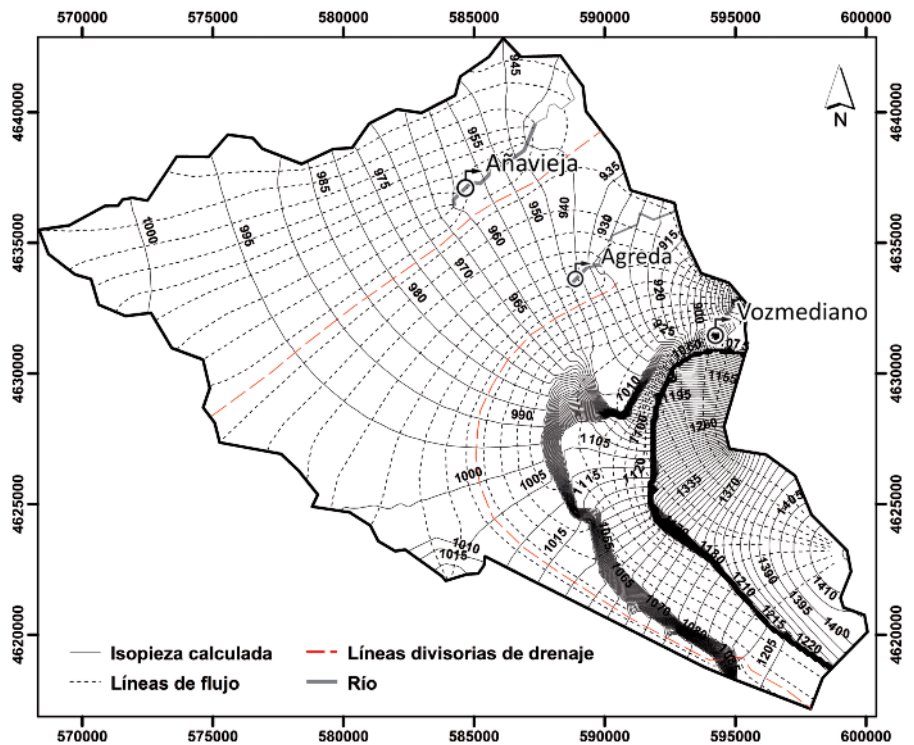
Fig. 3.-Modelo de drenaje del Macizo del Moncayo en su vertiente suroccidental; mapa de isopiezas calculado.
