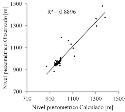
Fig. 2.- Nivel piezométrico observado y calculado.
