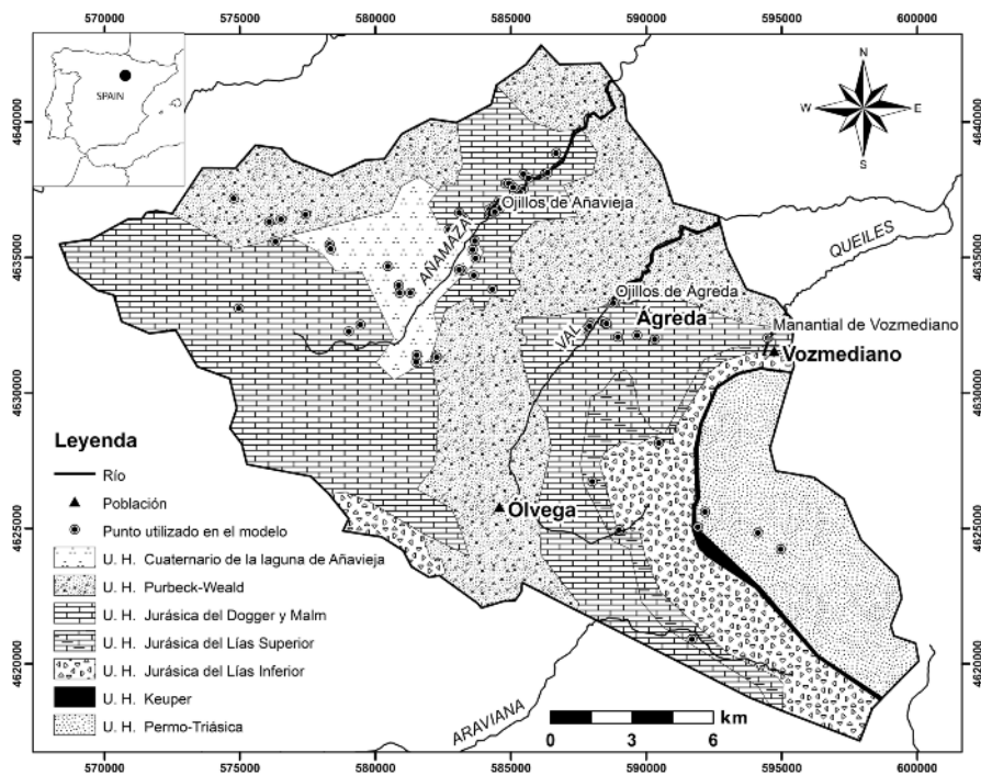
Fig. 1.- Localización geográfica de las zonas de estudio, zonificación del modelo y puntos de observación utilizados.
