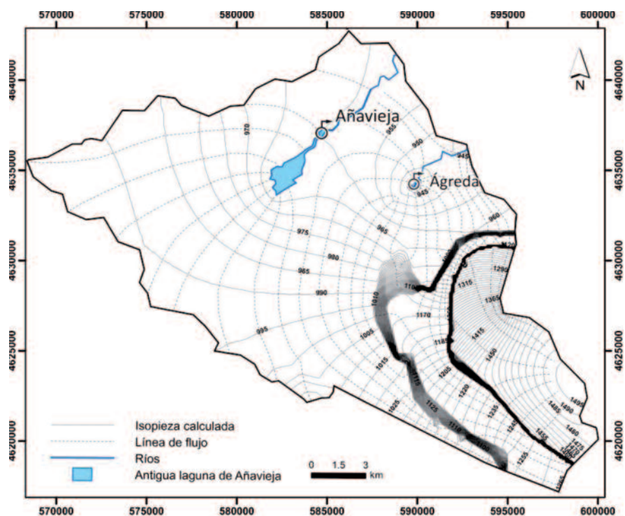
Fig. 4.- Mapa de isopiezas calculado sin el manantial de Vozmediano.
