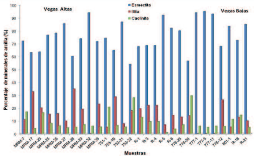
Fig. 3.- Distribución de los resultados semi-cuantitativos de los minerales de arcilla en la fracción < 2 μm, (asociación esmectita (predominante)-illita-caolinita, representativa de la SDS).
