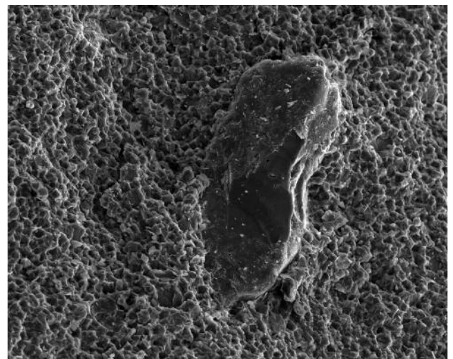
Fig. 4.- Grano de cuarzo rodeado por dolomita con tetura microesparítica.
