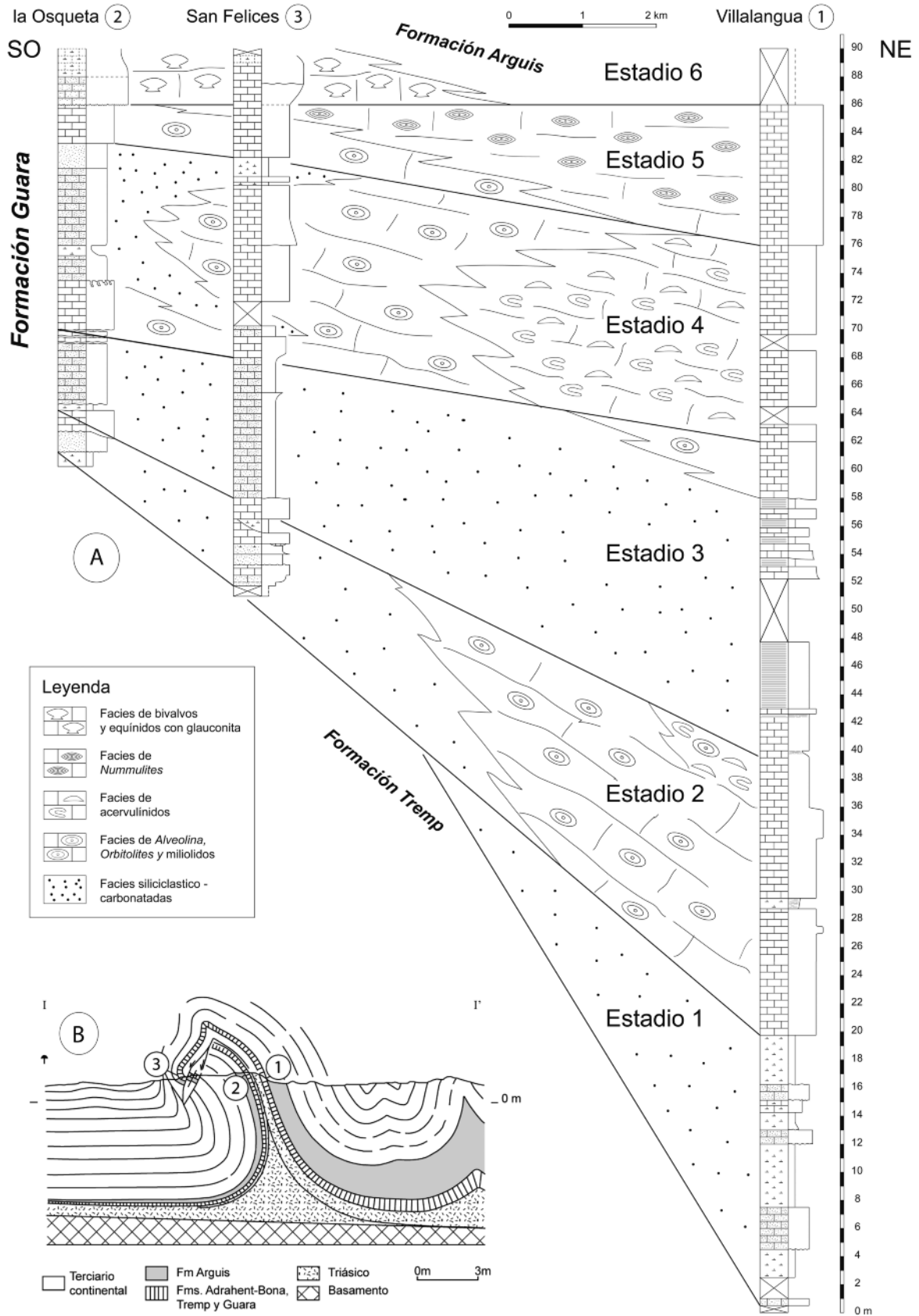
Fig. 2.- A. Panel de correlación de los perfiles estudiados. La situación de los perfiles, es el resultado de la restitución de la estructura de la Sierra de Santo Domingo. B. Corte geológico en el que se muestra la posición estructural de los perfiles estudiados (Villalangua, 1; la Osqueta, 2 y San Felices, 3), modificado de Millán et al. (1995).
