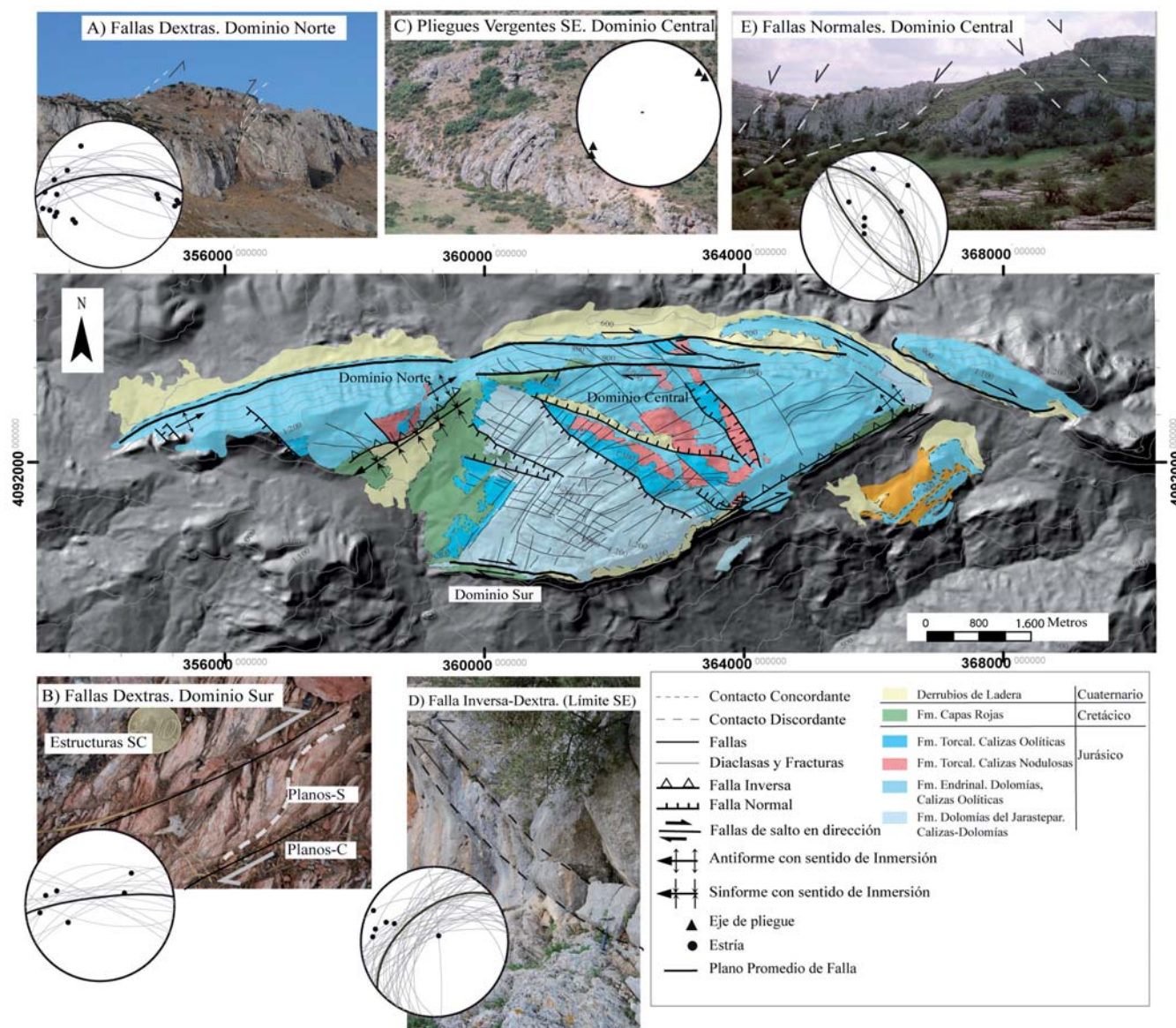
Fig. 2.- Mapa estructural del MTA (incorpora datos de IGME, 1991), en el que se muestran fotografías y diagramas de proyección equiareal (hemisferio inferior) de planos de fallas, estrias y ejes, correspondientes a algunas estructuras características: (A) fallas de salto en dirección dextro; (B) estructuras S-C asociadas a fallas de salto en dirección; (C) pliegues vergentes al SE; (D) fallas inversas y (E) fallas normales.
