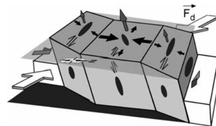
Fig. 3.- Modelo conceptual de la cinemática del MTA mostrando el reparto del flujo transpresivo en dominios estructurales. CSD: Dominio de cizalla simple en dirección. DC: Dominio de deformación coaxial.
