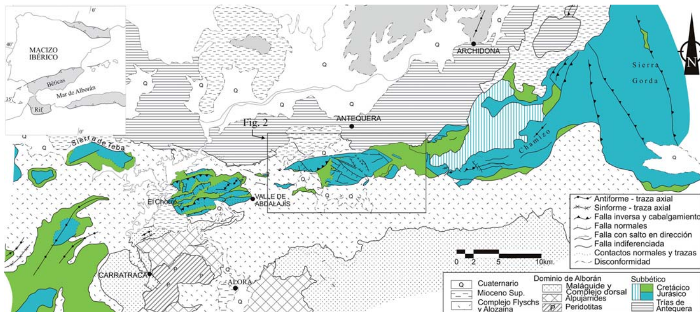
Fig. 1.- Mapa estructural de la zona de cizalla del Torcal y su localización en un marco tectónico regional. Fig. 1.- Structural map of the El Torcal shear zone and its location within the regional tectonic setting.
