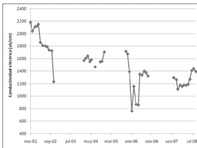
Fig. 8.- Variaciones de conductividad eléctrica desde 2001 a 2008. Pozo 29.
