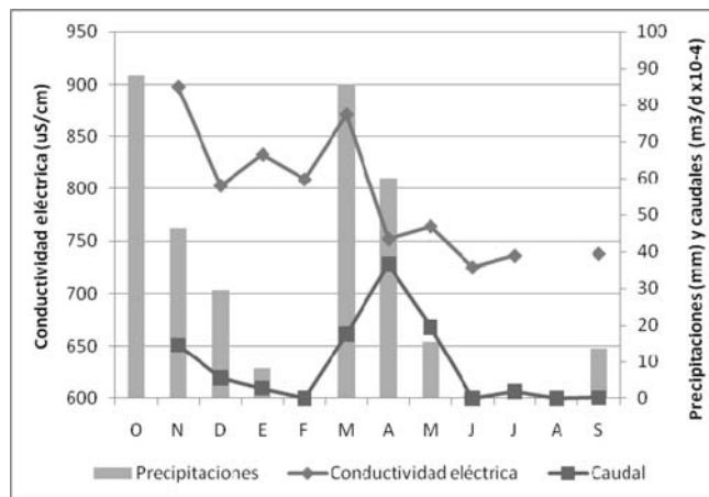
Fig. 6.- Variaciones de conductividad eléctrica. Pozo 7. 2001-2002.
