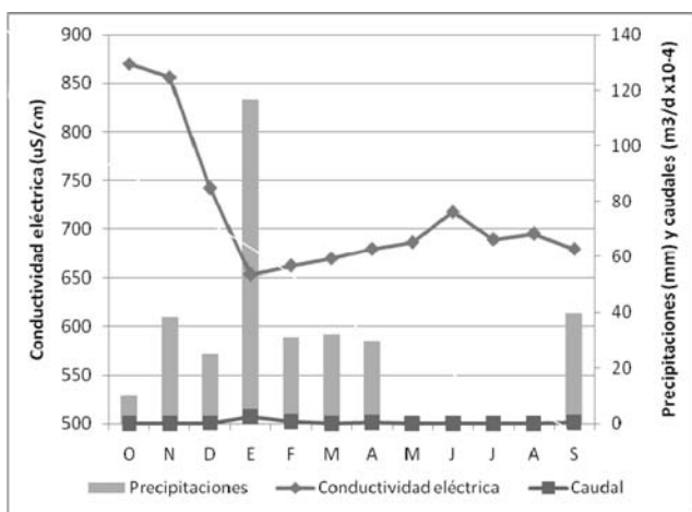
Fig. 7.- Variaciones de conductividad eléctrica. Pozo 7. 2005-2006.
