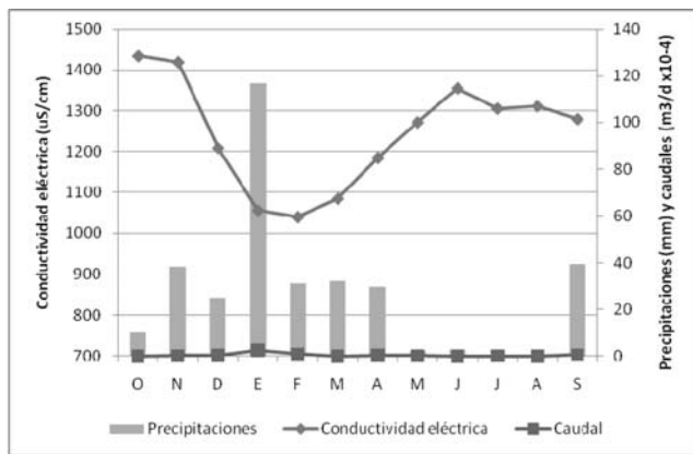
Fig. 5. Variaciones de conductividad eléctrica. Pozo 21. 2005-2006.
