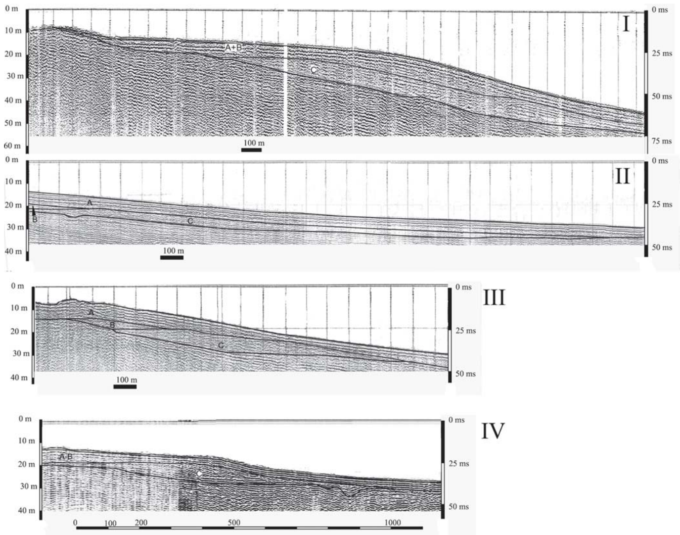
Fig. 2.- I) perfil sísmico «villaltea 1090-1123», II) perfil sísmico «Puigcampana 352-371», III) perfil sísmico «bahiaalicante 3313-3384» y IV) perfil «Santa 3188-3490». A) Sedimentos recientes ligados a la posición del nivel del mar actual en los últimos 6000 años BP. B) Sedimentos transgresivos debidos a la elevación del nivel del mar desde hace 8400 años hasta 6000 años BP. C) prisma sedimentario interpretado como formado durante el «evento 8.2 ka». Escala de profundidades en m a la izquierda y de tiempo doble a la derecha.
