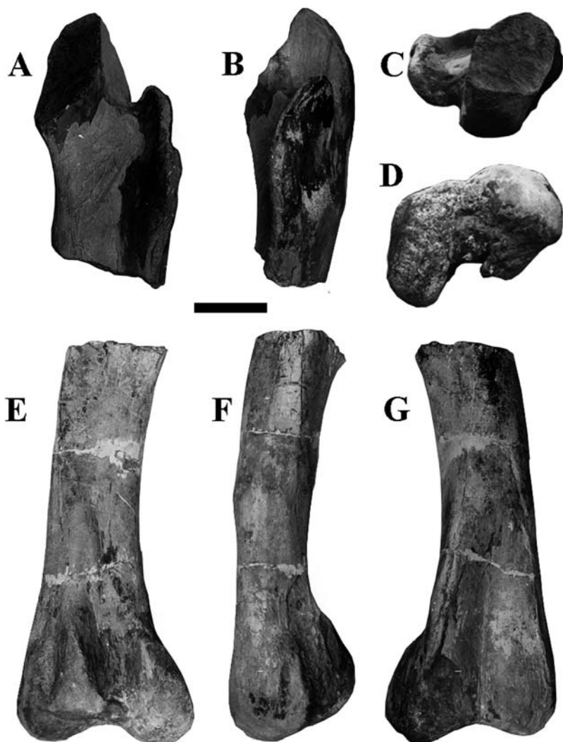
Fig. 1.- Fotografías realizadas por José Royo y Gómez (tomadas del documento ACN138/004) del fémur izquierdo atribuido a un terópodo tetanuro procedente del Cretácico Inferior de Morella. A-C: extremo proximal. D-G: extremo distal. A) vista anteromedial; B) vista posterior; C) vista proximal; D) vista distal; E) vista posterior; F) vista lateral; G) vista anterior. Escala 10 cm.
