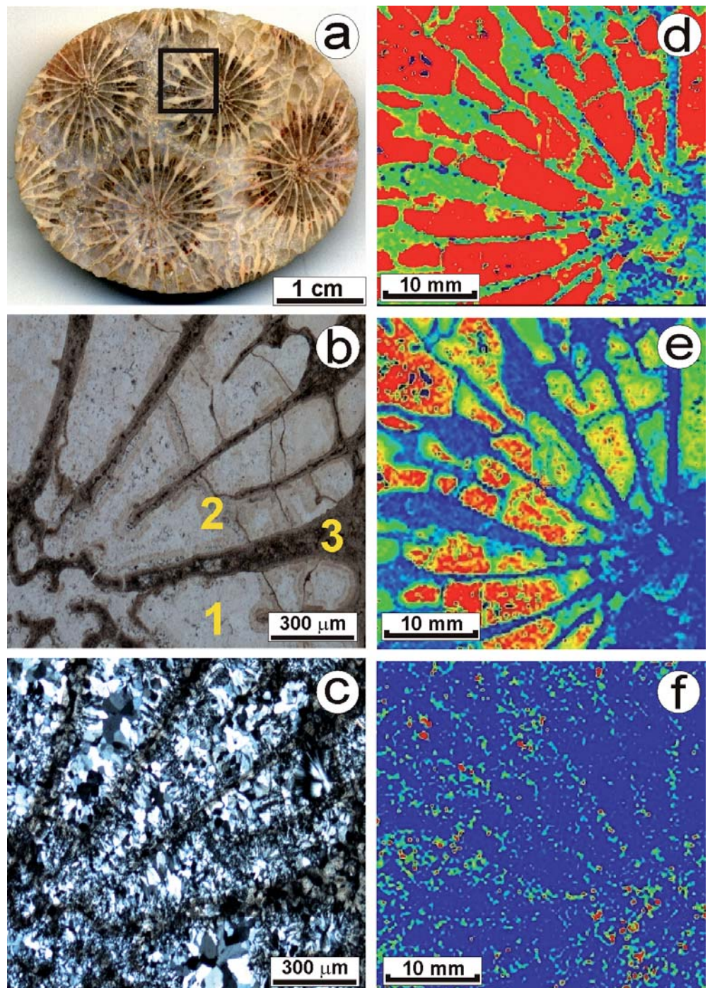
Fig. 3.- Imágenes de microscopía óptica (izquierda) y de Raman hiperespectral (derecha) de coral silicificado tomando la intensidad del pico 465\text{ cm}^{-1} como escala de referencia, (a) cabujón con señalización de la zona estudiada. (b) Texturas de la sílice en MOP con nícoles paralelos, indicando con 1,2, y 3, las tres zonas descritas en el texto. (c) Idem con nícoles cruzados. (d) Imagen Raman, donde se observan los contrastes en verde y azul para las zonas de baja cristalinidad de la sílice, y en rojo para el cuarzo. (e) Ídem para las zonas de alta cristalinidad mostrando en azul las partes poco cristalinas, y en rojo-amarillo-verde de más a menos cristalinidad. (f) Distribución de las partículas de materia carbonácea en rojo, principalmente en las septas y en el núcleo central.
