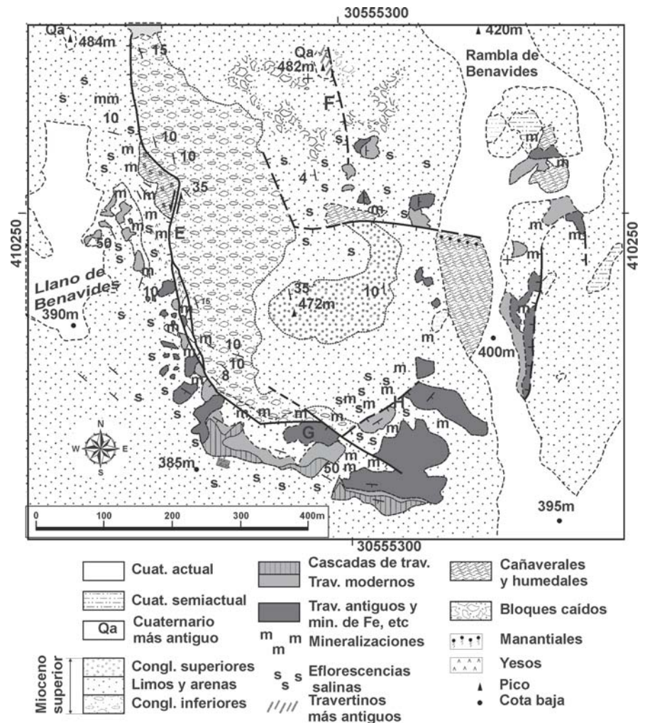
Fig. 4.- Esquema geológico de los travertinos del sector de Benavides. Su situación puede verse en la Fig. 1 B. Las letras E a H indican la posición de las fotos de la Fig. 5.
