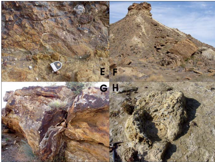
Fig. 5.- Foto E: Detalle de la principal falla del sector de Benavides. Las falla es normal sinistrorsa y las estrías se hunden hacia la derecha. Foto F: Los travertinos más antiguos en la cota 482. Pueden verse numerosos bloques caídos a su alrededor. Foto G: Travertinos mineralizados en el sector de Benavides. Foto H: Estructura aproximadamente circular correspondiente a un punto de salida de agua. Se ha marcado uno de los círculos. Los asteriscos señalan la posición de tubitos con óxidos de hierro que se ven como puntos oscuros.
