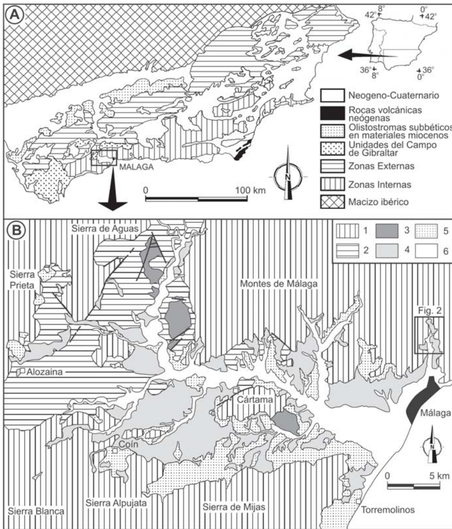
Fig. 1.- Localización de la cuenca de Málaga en el ámbito de la Cordillera Bética (A) y mapa geológico de la cuenca (B). 1: Zona Interna (complejo Alpujarride y Maláguide); 2: Complejo del Campo de Gibraltar; 3: Tortonense; 4: Plioceno inferior; 5: Cuaternario; 6: Depósitos fluviales recientes.
