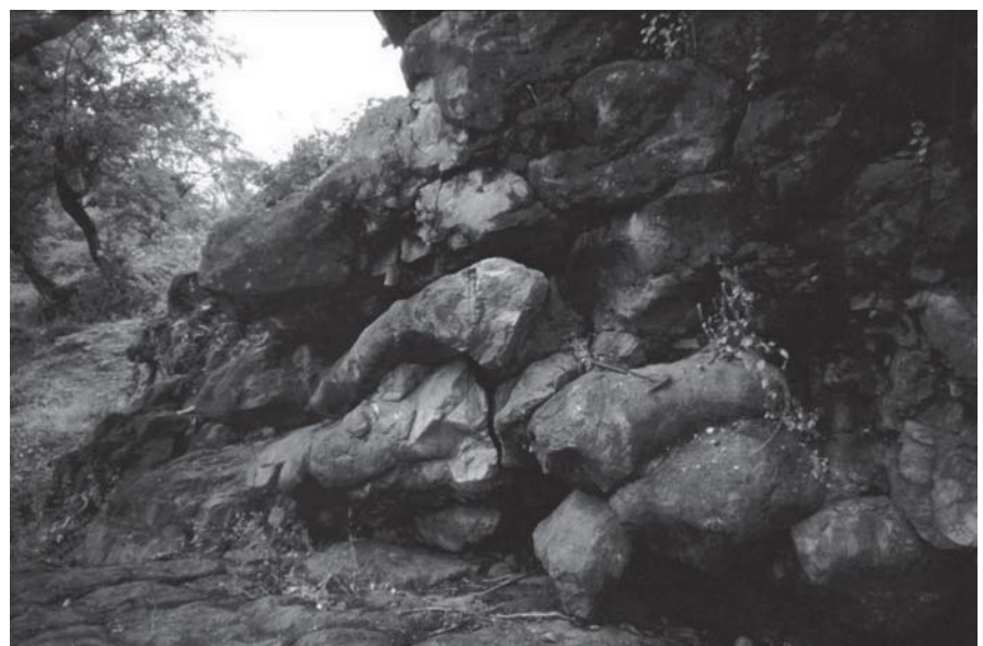
Fig. 3.- Basaltos Toléiticos Almohadillados del Grupo Basal Volcánico (GBV).
