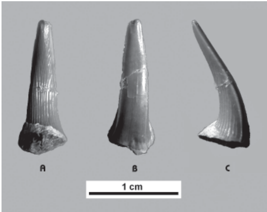
Fig. 3.- Diente de Scapanorrhynchus raphyodon (Agassiz) en vistas a) lingual, b) labial y c) lateral.
