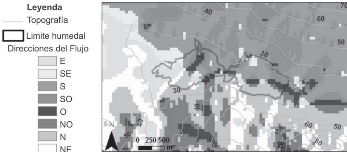
Fig. 3.- Mapa de dirección del flujo
