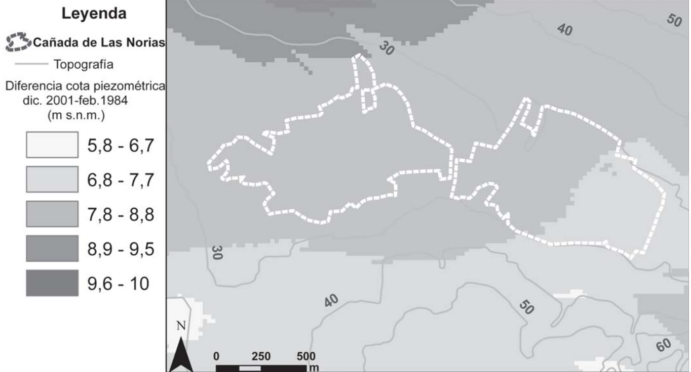
Fig. 5.- Variación piezométrica entre los años 1984 y 2001 (m s.n.m.)
