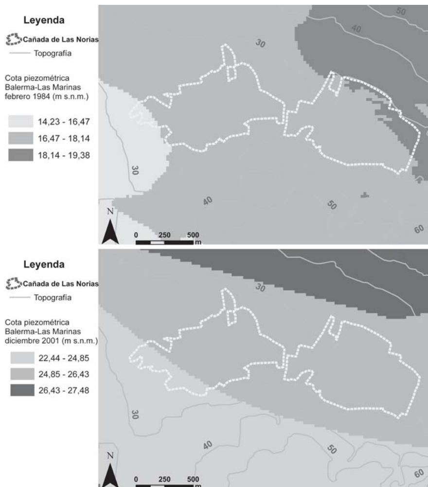
Fig. 4. - Mapas piezométricos (m s.n.m.) del acuífero de Balerma-Las Marinas (Febrero 1984 y Diciembre 2001)
