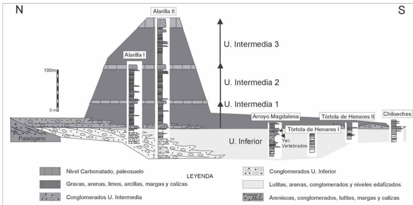
Fig. 2.- Correlación estratigráfica.
