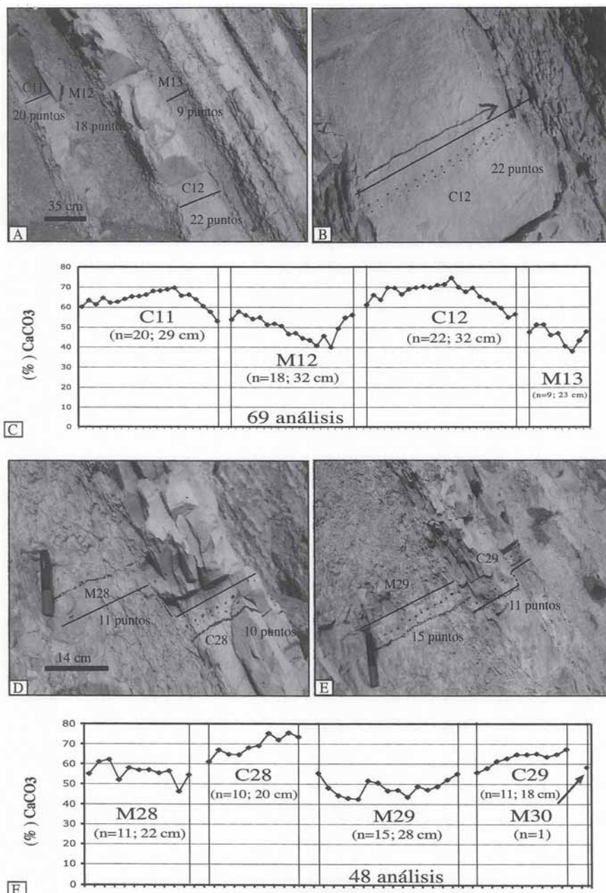
Fig. 3.-Detalle de los lechos analizados y variaciones del (%) CaCO 3 en alta resolución. Explicaciones en el texto.
