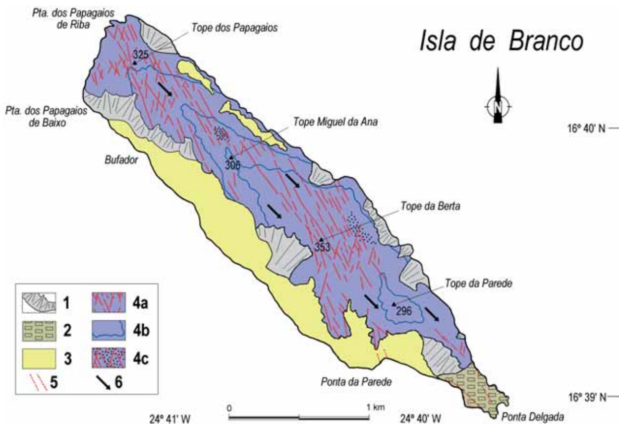
Fig. 4.- Mapa geológico de la isla de Branco. 1: coluviones; 2: rasa; 3: arenas eólicas; 4: coladas y piroclastos basálticos: 4a: diques, 4b: capas guía, 4c: áreas con piroclastos abundantes; 5: diques parcialmente cubiertos; 6: inclinación de las coladas.
