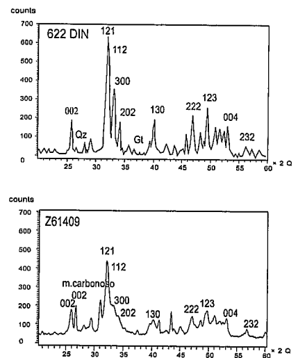
Fig. 2.- Difractograma de fósiles de huesos procedentes de Zambrana (A) y Laño (B). El componente mineral mayoritario de las muestras es la francolita, con pequeños picos pertenecientes a cuarzo (Qz) y goethite (Gt).
