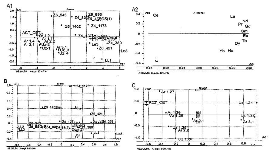
Fig. 4.- Análisis de componentes principales de tierras raras. En A1 aparecen los scores de todas las muestras, incluyendo las del yacimiento de Laño (tomadas de Lecuyer et al. , 2003); A2, loadings. Pueden diferenciarse dos grupos de muestras, tratados individualmente en las figuras B (muestras de Laño y Zambrana) y C (muestras de Ardanatz, Uztarrotz y actuales).
