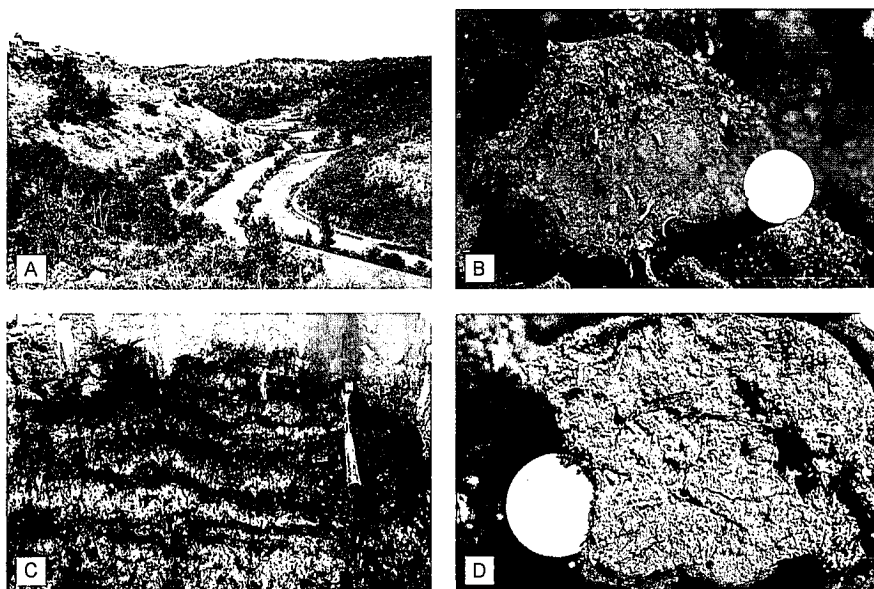
Fig. 3.- 3A/ Panorámica del valle del río Ugría a la altura de Fuentes de La Alcarria. 3B/ Detalle de Turba con restos vegetales de dos tipos, los primeros de colores más claros con estructura vegetal manifiesta y los segundos de menor tamaño y dispuestos a modo de matriz. 3C/ Turba alternando con margocalizas blanquecinas. A techo margas grises. 3D/ Detalle de margocalizas con indicios de restos vegetales.
