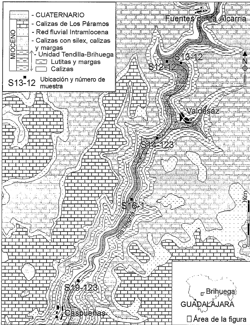
Fig. 1.- Mapa Geológico y de situación de muestras. Modificado a partir de Aznar et al. (1990).
