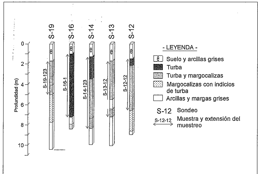
Fig. 2.- Perfiles de sondeos.
