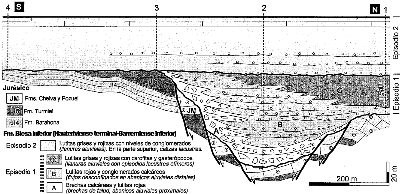
Fig. 2.- Distribución de facies en la Fm. Blesa (parte inferior).
