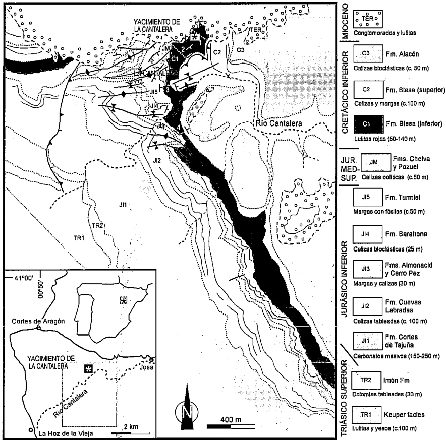
Fig. 1.- Cartografía geológica del entorno del yacimiento de La Cantalera.
