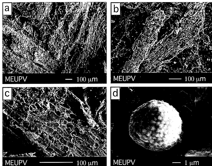
Fig. 2.- Imágenes de SEM: a) restos de tallos con aspecto leñoso; b) fragmentos alargados con microestructura celular interna bien definida; c) detalle de los fragmentos anteriores donde se aprecia el contorno poligonal de las células; d) framboides de piritita en el interior de una celdilla de la concha de un rudista radiolítido.
