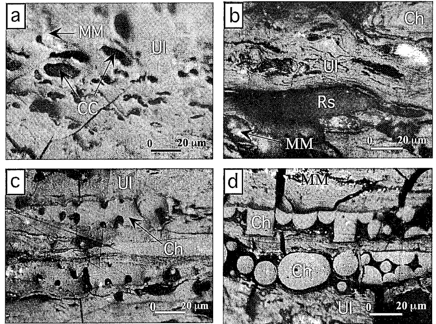
Fig. 3.- Microfotografías de la materia orgánica (MM: materia mineral; Ul: ulminita; Ch: corpohuminita; Rs: resinita; CC: cavidades celulares): a) detalle del tejido vegetal (ulminita) con las cavidades celulares abiertas, vacías o rellenas por materia mineral oxidada; b) detalle del tejido vegetal (ulminita) algo menos gelificado, mostrando la microestructura de las paredes. Las cavidades celulares aparecen abiertas o semicerradas, y rellenas por resinita y/o materia mineral alterada. Se observa la corpohuminita con una reflectancia ligeramente más elevada que la de la ulminita; c) la corpohuminita muestra una porosidad importante; en cambio, la ulminita presenta un mayor grado de gelificación; d) corpohuminita con estructura tabular, esférica y subsférica. Se desarrollan grietas y fracturas por alteración. El tejido vegetal se encuentra bastante gelificado y la materia mineral se entremezcla con el material orgánico.
