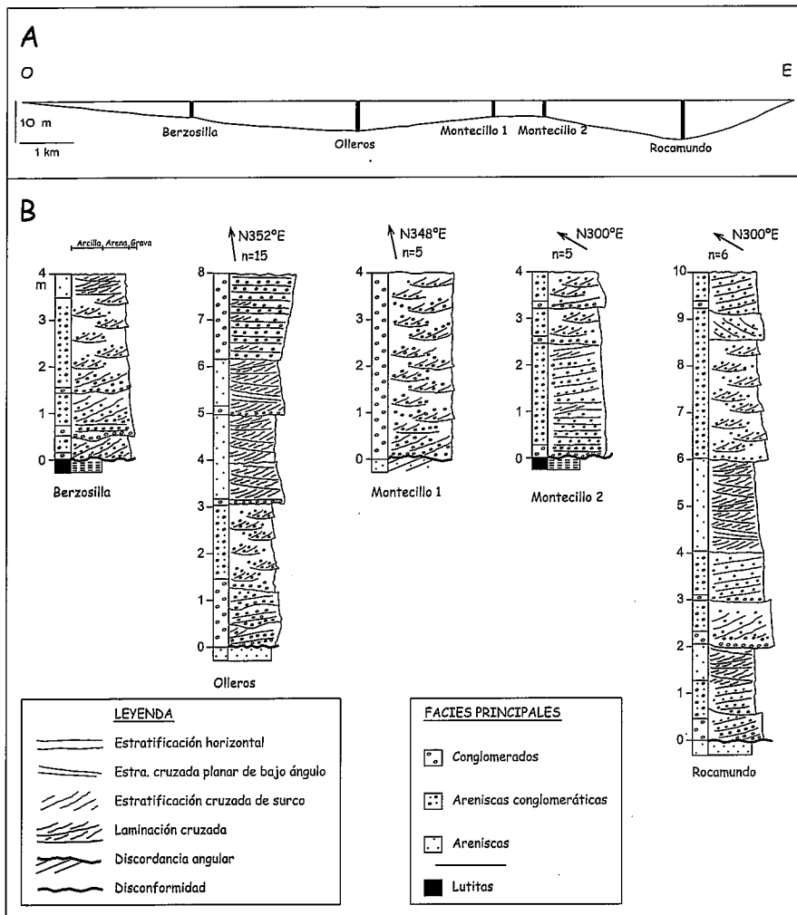
Fig. 2.- A: Geometría de la unidad de La Iglesia de Olleros (escala vertical x 80) disposición espacial de las columnas. B: Características litológicas y facies principales.
