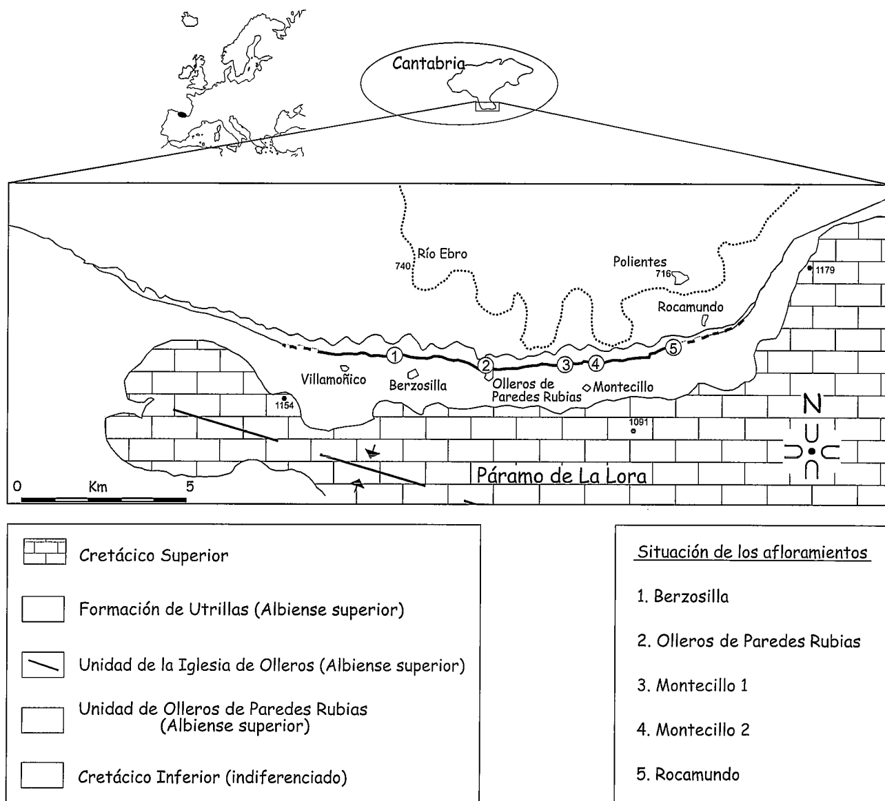
Fig. 1.-Localización geográfica y geológica del área de estudio con situación y topónimos de las columnas realizadas.
