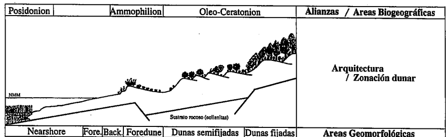
Fig. 2.- Modelo de zonación de los sistemas dunares en la bahía de Alcudia.
