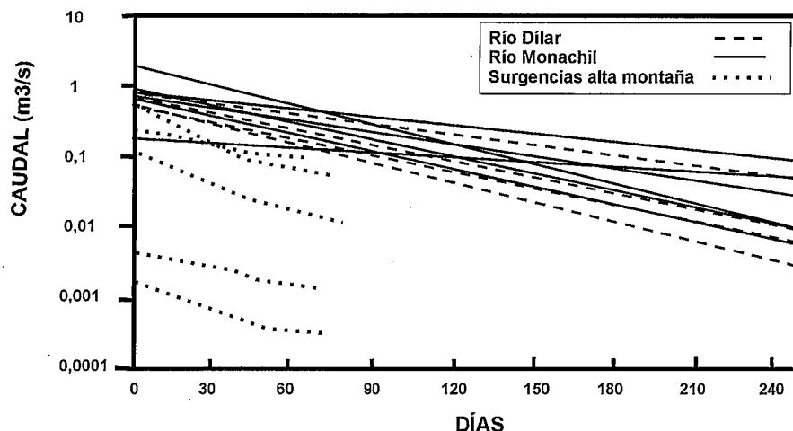
Fig. 3.- Curvas de agotamiento, en escala semilogarítmica, obtenidas para los ríos Dílar y Monachil y para surgencias de la franja glaciar y periglacial
