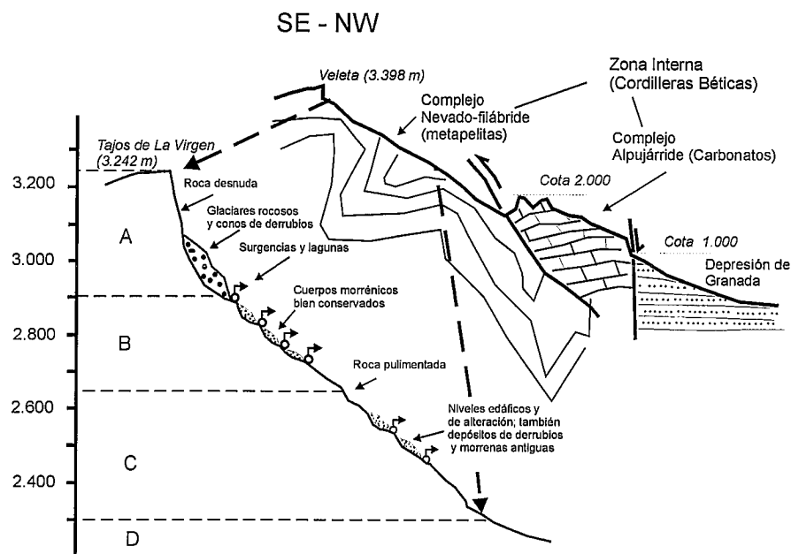
Fig. 2.- Croquis simplificado con las diferentes franjas hidrológicas altitudinales que se pueden distinguir en la cuenca del río Dílar (3.242 a 2.300 m de altitud)
