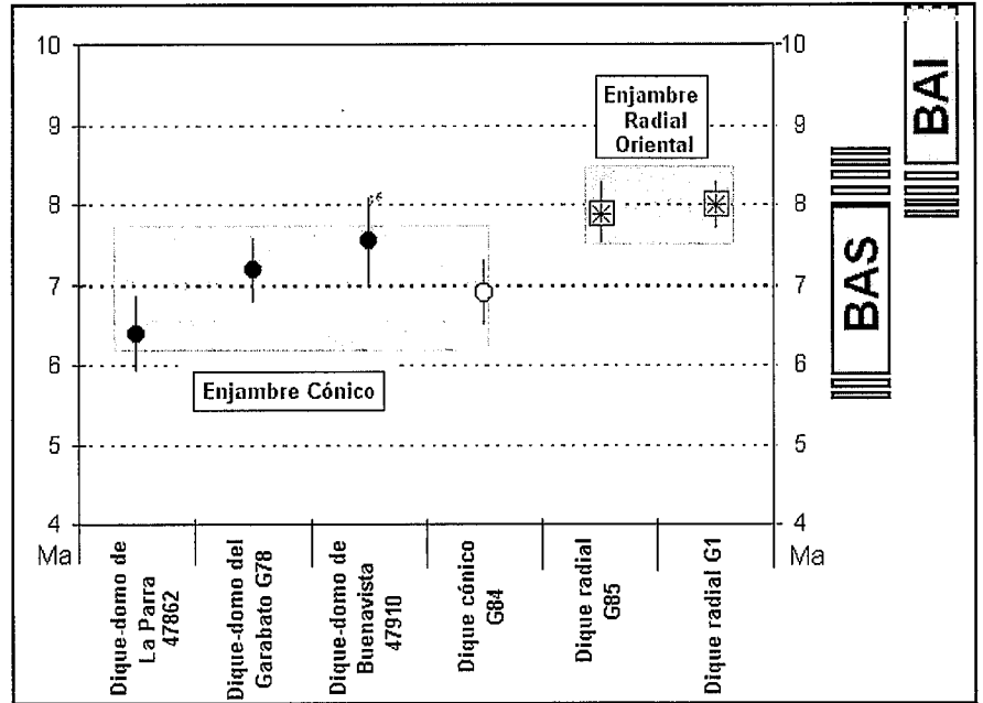
Fig. 2: Edades radiométricas K/Ar de los diques sálicos en relación con los Basaltos Antiguos Inferiores (BAI) y los Basaltos Antiguos Superiores (BAS).
