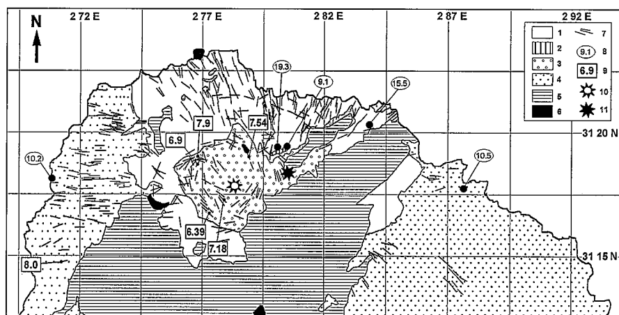
Fig. 1: Esquema geológico del Norte de la isla de La Gomera y distribución de los diques sálicos. 1: Complejo Basal; 2: Sienitas de Tamargada; 3: Complejo Traquítico-Fonolítico; 4: Basaltos Antiguos; 5: Basaltos Subrecientes; 6: Domos sálicos de la serie de Los Roques; 7: Diques sálicos; 8: Edades K/Ar (Ma) publicadas en trabajos anteriores; 9: Edades K/Ar (Ma), este trabajo; 10: centro del enjambre cónico de Vallehermoso y del enjambre radial occidental; 11: Centro del enjambre radial oriental.
