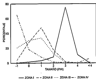
Figura 6- Curvas de frecuencia relativa de las distribuciones granulométricas características de las zonas diferenciadas.
