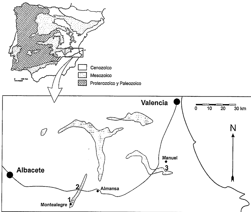
Figura 1: Situación de las secciones estratigráficas muestreadas en este estudio. 1, Sección de Montealegre (norte del pueblo); 2, Sección de Almansa (corte de la carretera); 3, Sección de Manuel (sur del pueblo). En gris los principales afloramientos del Keuper.
