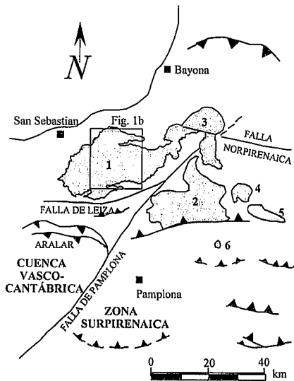
Fig.2. Macizos paleozoicos en el NO de Los Pirineos (1: Macizo de Cinco Villas; 2: Macizo de Quinto Real). Modificado de Martínez-Torres, 1997
