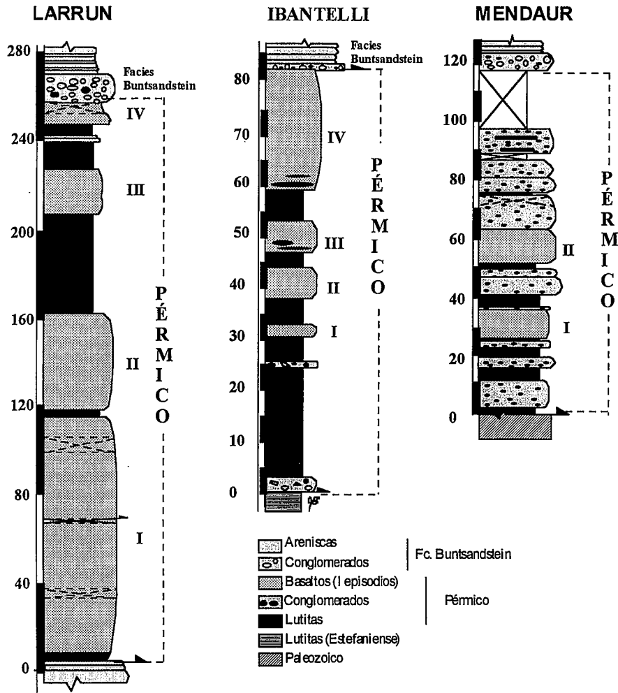
Fig.5. Columnas estratigráficas en los tres sectores con afloramientos de basaltos.
