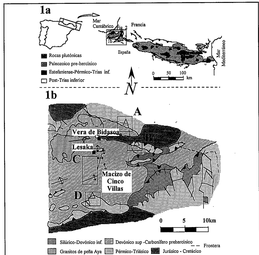
Fig.1. Situación de la zona de estudio: 1a) En el contexto pirenaico; 1b) de los sectores estudiados (A: Larrun; B: Ibantelli; C: Yanci-Aranaz; D: Mendaur).
