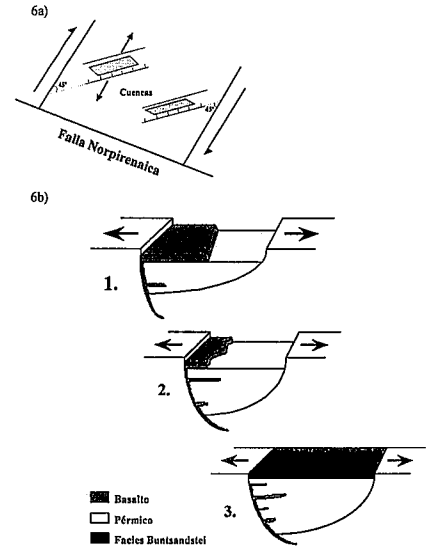
Fig. 6. Formación de las cuencas; 6a) En el contexto paleogeográfico del Pérmico superior; 6b) evolución de las cuencas.
