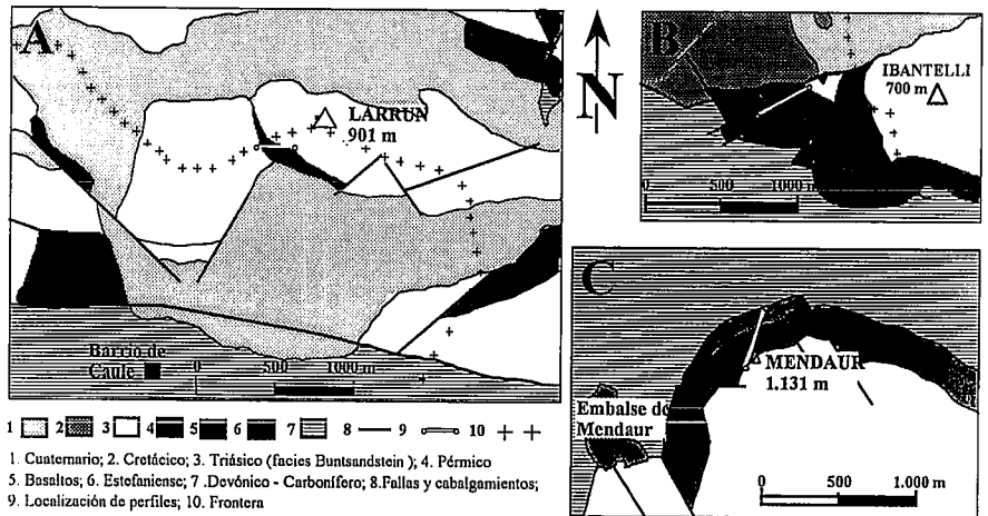
Fig. 3. Esquema geológico de los sectores estudiados en basaltos. (A: Larrun; B: Ibantelli; C: Mendaur. Se indica la situación de las columnas de Fig.5.
