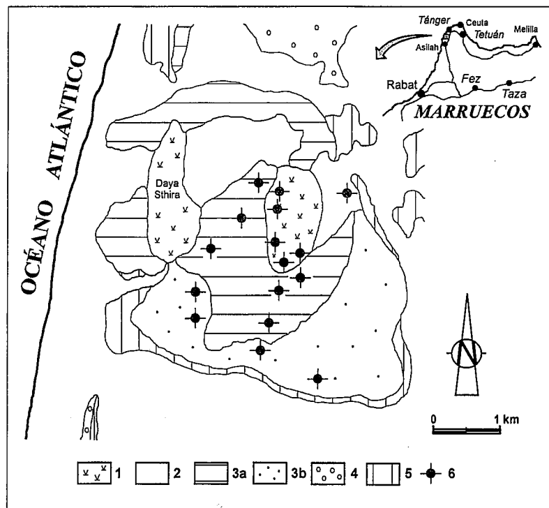
Fig. 1.- Localización geológica y esquema hidrogeológico del área de estudio. 1: humedales; 2: Cuaternario; 3: Neógeno (a: Mioceno superior -formación inferior-; b: Plioceno); 4: areniscas numídicas; 5: Unidad de Tánger; 6: sondeo.
