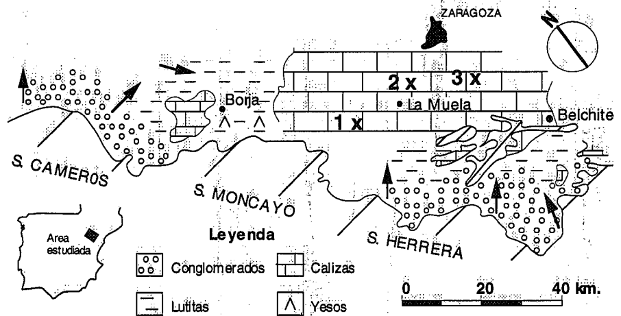
Fig. 1.- Esquema de situación y distribución de facies durante el Mioceno medio en el sector central de la Cuenca del Ebro. X: Situación de perfiles. 1: La Muela Sur, 2: La Muela Norte, 3: La Plana.
