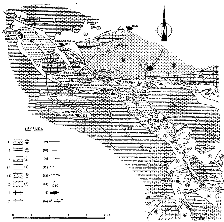
Fig. 1.- Esquema geológico del polje de Conquezueta-Ambrona-Torralba (después de las cartografías geológicas de Bascones y Martínez 1981; Adell et al. , 1981, 1982; Lendínez 1991 y datos propios). Leyenda 1: margas, arenas y conglomerados; 2: arenas, calizas, margas y dolomías; 3: calizas, dolomías, carniolas y margas; 4: margas y yesos; 5: dolomías y margas; 6: conglomerados, areniscas y arcillas; 7: anticlinal; 8: sinclinal; 9: falla; 10: dirección e inclinación de capas; 11: contacto normal; 12: contacto discordante; 13: cauces con dirección y sentido del flujo; 14: cota en metros; 15: núcleo urbano; 16: yacimientos arqueológicos de Miño, Torralba y Ambrona; B: Buntsandstein; M: Muschelkalk; K: Keuper; J: Jurásico; C: Cretácico; Q: Cuaternario.
