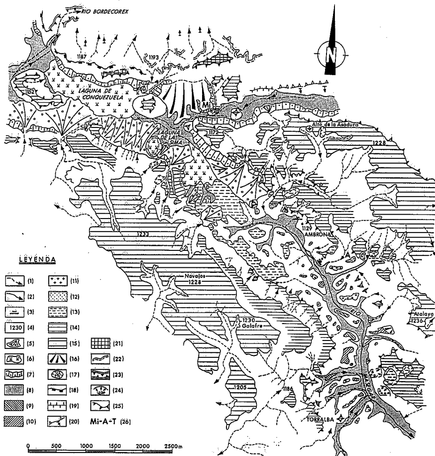
Fig. 2.- Mapa geomorfológico del sector central y meridional del polje de Conquezuella: valles de los ríos Bordecorex y Masegar. Leyenda. 1: flujo episódico/estacional; 2: flujo permanente; 3: manantial; 4: cota en metros; 5: cono aluvial; 6: laguna; 7: coluvión; 8: llanura aluvial; 9: terraza a +7-9 m; 10: terraza a +15 m; 11: terraza a +22 m; 12: terraza a +35 m; 13: Superficie de Ambrona (S.A.); 14: Superficies M1 y M2, no diferenciadas; 15: Superficie M3; 16: glacis; 17: dolina; 18: cornisa en arenisca; 19: barra en dolomía; 20: monoclinales; 21: replano estructural; 22: relieve ruiforme; 23: cañón; 24: movimiento de masa; 25: talud/escarpe; 26: yacimientos arqueológicos de Miño, Ambrona y Torralba.
