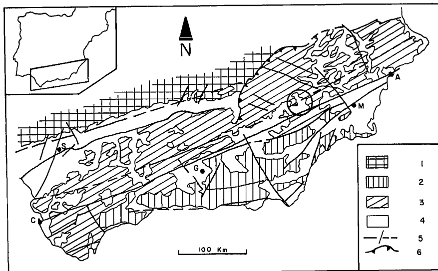
Fig. 1.- Mapa geológico esquemático de las Cordilleras Béticas (SE de España). El círculo marca la localización de la Cuenca de Caravaca. 1: Macizo Ibérico; Cordilleras Béticas, 2: Zonas Internas; 3: Zonas Externas; 4: Cuencas Neógenas; 5: Trazas de las principales fallas (y trazas probables); 6: Límite de antepaís; A: Alicante; M: Murcia; G: Granada; S: Sevilla; C: Cádiz. Simplificado de Baena et al. (1994).
