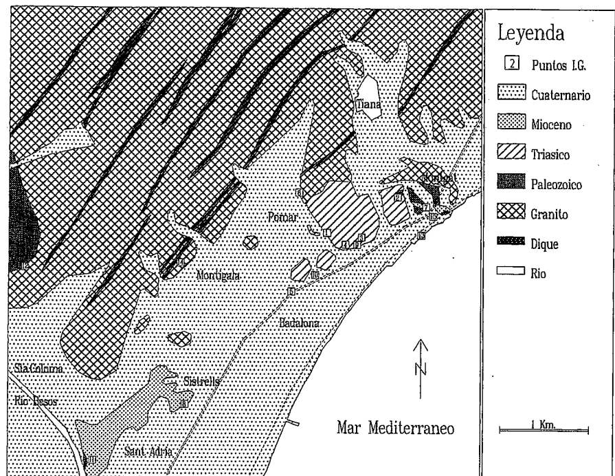
Esquema Geológico de Badalona
