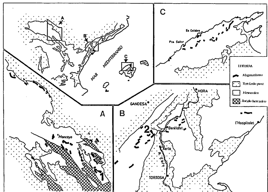
Fig.1. Localización del magmatismo alcalino en tres sectores del borde nord-oriental de la Península Ibérica (A: borde NO de la Cadena Ibérica, B: Cadenas Costero Catalanas en Tarragona y C: Sierra Norte de Mallorca).
