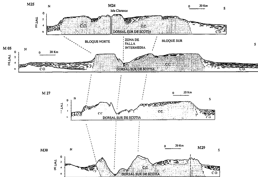
Fig. 2.- Esquema interpretativo de los perfiles sísmicos que muestran los rasgos tectónicos principales de los perfiles transversales a la Dorsal Sur de Scotia. C.C., Corteza continental. C.O., Corteza oceánica. Las líneas discontinuas indican la correlación de los rasgos tectónicos principales.
