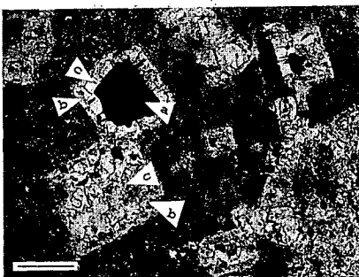
Fig. 6.- Piritas (a) precipitadas en la matriz que están sustituidas en gran parte por clorita (b) y carbonato cálcico que sustituye a ambos (c). Barra de escala: 0,4mm
