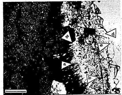
Fig. 5.- Estilolito (E) desarrollado en el contacto de la matriz con los cementos radiaxiales de la septaria (a). b) Cemento de calcita de aspecto sucio. c) Piritas. d) Cuarzo. e) Calcita en diente de perro. Barra de escala: 0,2mm
