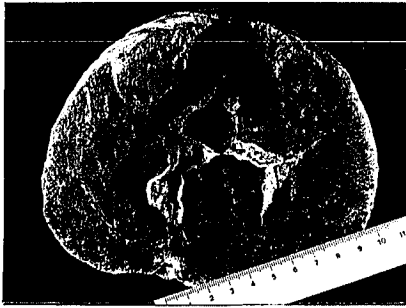
Fig. 2.- Concreción carbonatada septarizada en la que se aprecia la distribución de las septarias y algunos cementos que las rellenan. Barra de escala en centímetros.
