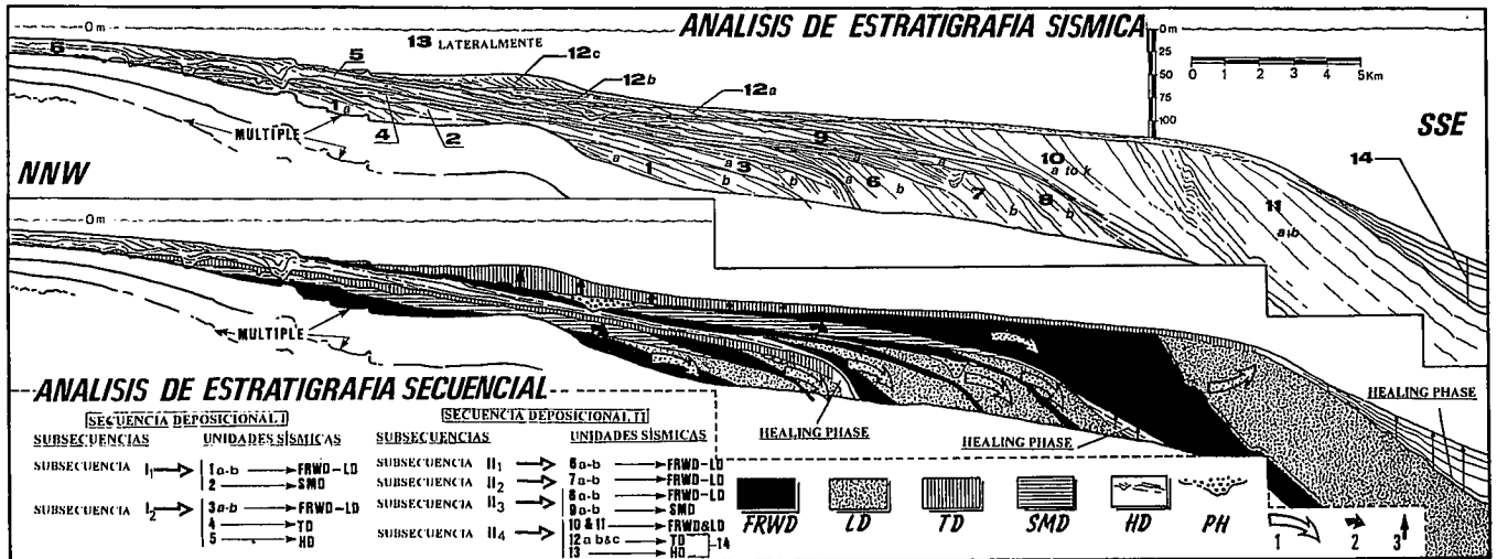
Fig. 2.- Interpretación del perfil sísmico de alta resolución (Geopule. 175 J) mostrando las unidades sísmicas y las secuencias deposicionales. FR FRWD: depósitos regresivos; LD: depósitos de bajo nivel; TD: depósitos transgresivos; SMD: depósitos de margen de plataforma, HD: depósitos de alto nivel; ph: paleocanales. 1.- progradaciones mayores; 2.- progradaciones menores & aggradación; 3.- aggradación. Localización en la figura 1.
