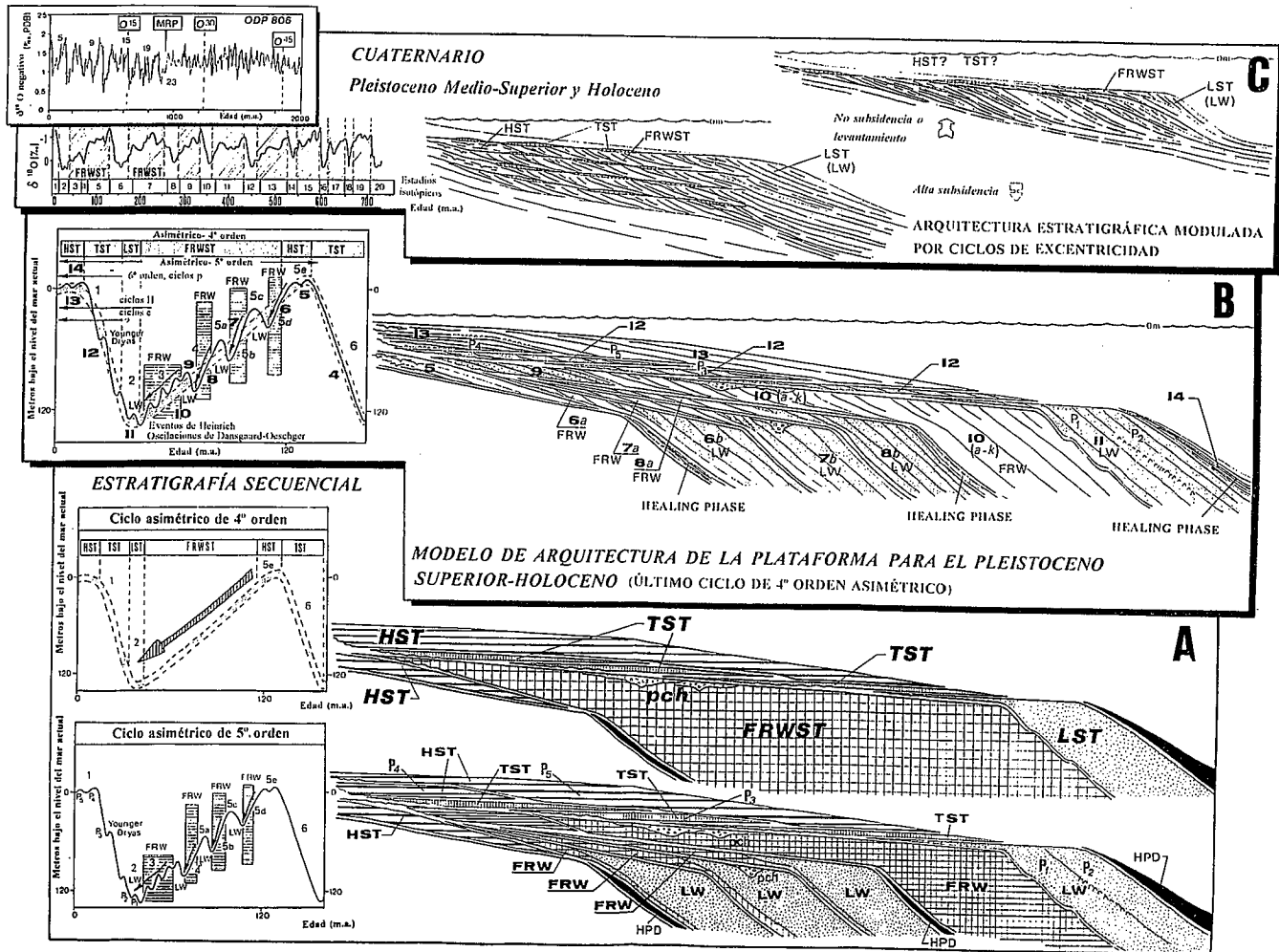
Fig. 3.- Modelo teórico sísmo-secuencial de alta resolución de la arquitectura de la plataforma continental, considerando ciclos eustáticos de diferente frecuencia que se modulan entre sí. A) Secuencia deposicional de 4º orden y geometría de los cortejos sedimentarios para los últimos 120.000 años B.P.; B) Secuencias deposicionales de 5º orden y geometría de los cortejos sedimentarios asociados. Se muestra la posición de las unidades sísmicas diferenciadas; C) Con posterioridad a la Revolución Climática del Pleistoceno Medio (MPR) la geometría de las secuencias deposicionales de 4º orden estructuran la plataforma continental mediante ciclos asimétrico de 100.000-120.000 años B.P caracterizados por suaves y graduales descensos del nivel del mar, bruscas subidas, y muy breves intervalos de alto nivel. La estructuración de las secuencias de cuarto orden esta profundamente condicionada por las características particulares de la subsidencia de cada margen continental. En un margen con una elevada subsidencia la estructuración de las secuencias sera vertical y por tanto agradante, mientras que en un margen sin subsidencia o incluso levantamiento, la estructuración de las secuencias sera lateral, y por lo tanto progradante.
