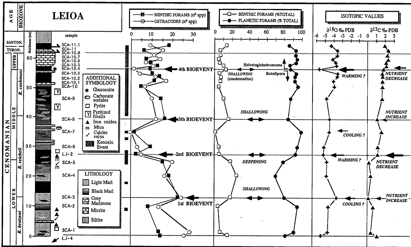
Fig. 2. Evolución de los parámetros bióticos (foraminíferos, ostrácodos) e isotópicos ( \delta^{13}\text{C} , \delta^{18}\text{O} ) en la serie de Leioa (Bizkaia) durante el Cenomaniense. Se definen cuatro bioeventos caracterizados por la variación de los mencionados parámetros.
