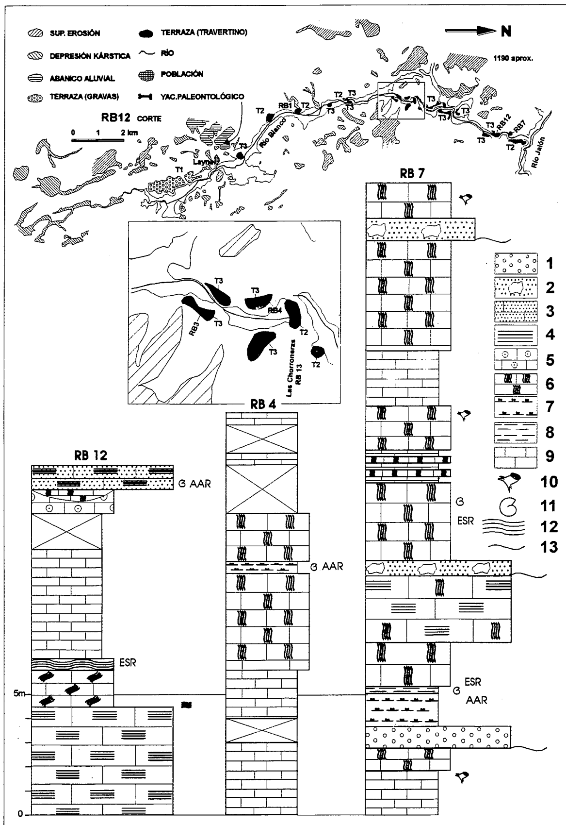
Fig. 1.- Esquema geomorfológico y columnas estratigráficas A (RB-4 nivel antiguo), B (RB-7, nivel intermedio), C (RB-12, nivel más reciente). 1-gravas, 2-bloques y arena, 3-travertino de intraclastos, 4-t. de fitoclastos, 5-t. con oncolitos, 6-t. con tallos en posición de vida, 7-limolitas, 8-arcilla, 9-t. micrítico, 10-moldes de troncos, 11-gasterópodos, 12-laminación algal, 13-discordancia.
