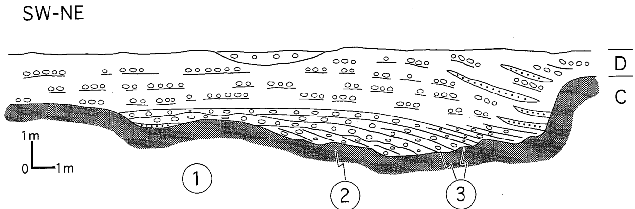
Fig. 3.- Esquema de un tramo con acreción lateral en un canal conglomerático. C) incisión inicial; D) colmatación y ensanche. Nótese las superficies convexas de acreción lateral. Misma numeración que en la figura 2.
