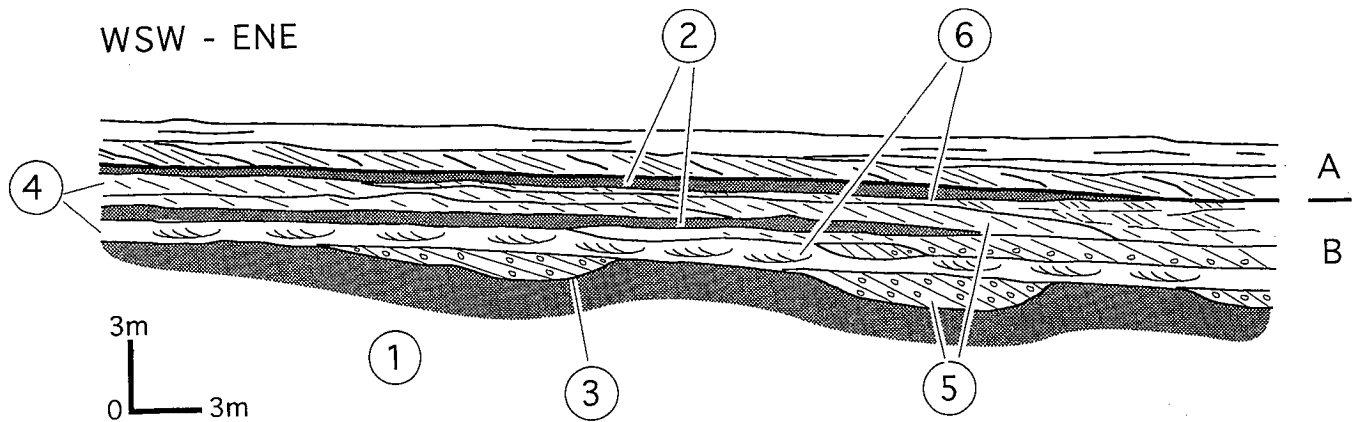
Fig. 2.- Esquema de los tramos rectilíneos. 1) depósitos de intercanal; 2) lutitas intercaladas; 3) facies de ocupación; 4) facies de desarrollo; 5) barras; 6) dunas. A) unidad superior; B) unidad inferior.
