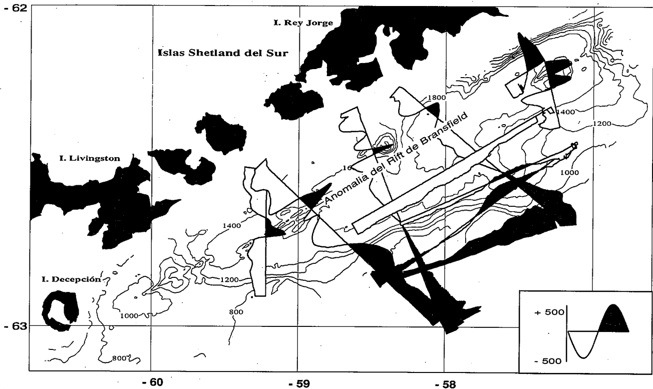
Fig. 4.—Perfiles de anomalías magnéticas registradas en la Cuenca Central de Bransfield.
