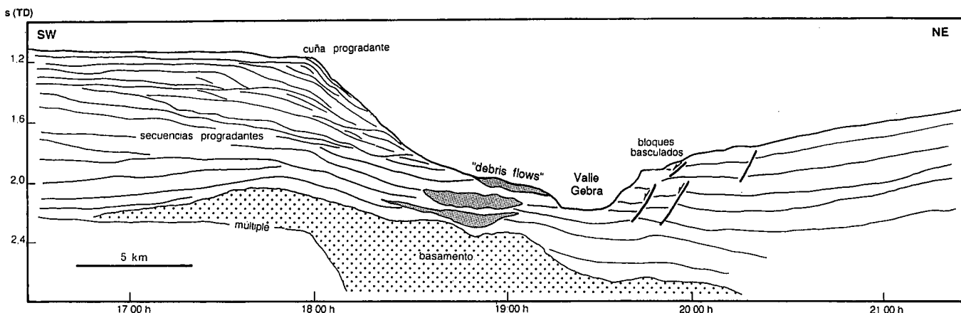
Fig. 3.— Perfil sísmico G7. Véase situación en la Fig. 1.
