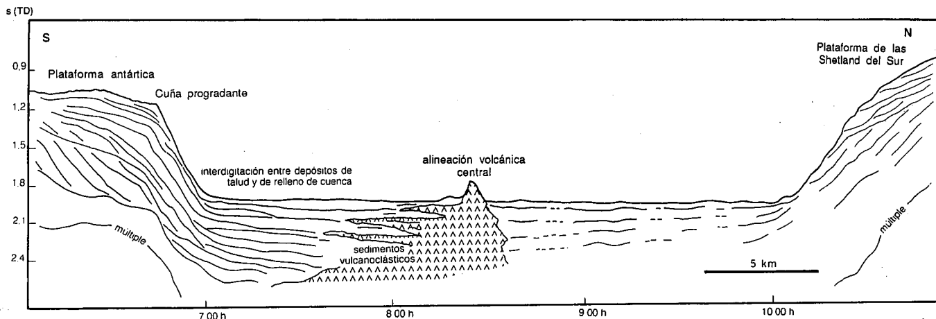
Fig. 2.— Perfil sísmico G1. Véase situación en la Fig. 1.
