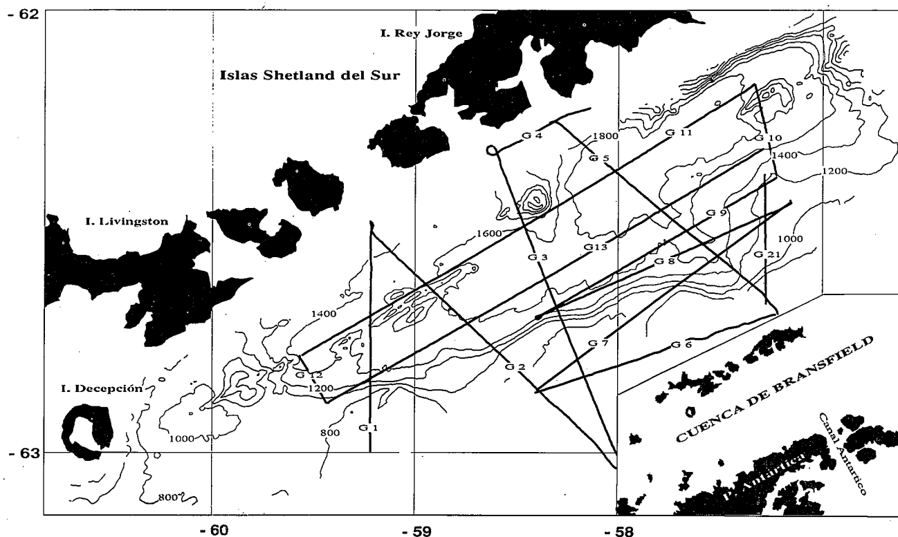
Fig. 1. — Situación de los perfiles de sismica de reflexión y de magnetismo sobre el esquema batimétrico de la Cuenca Central de Bransfield basado en los datos de multihaz de GEBRA '93.
