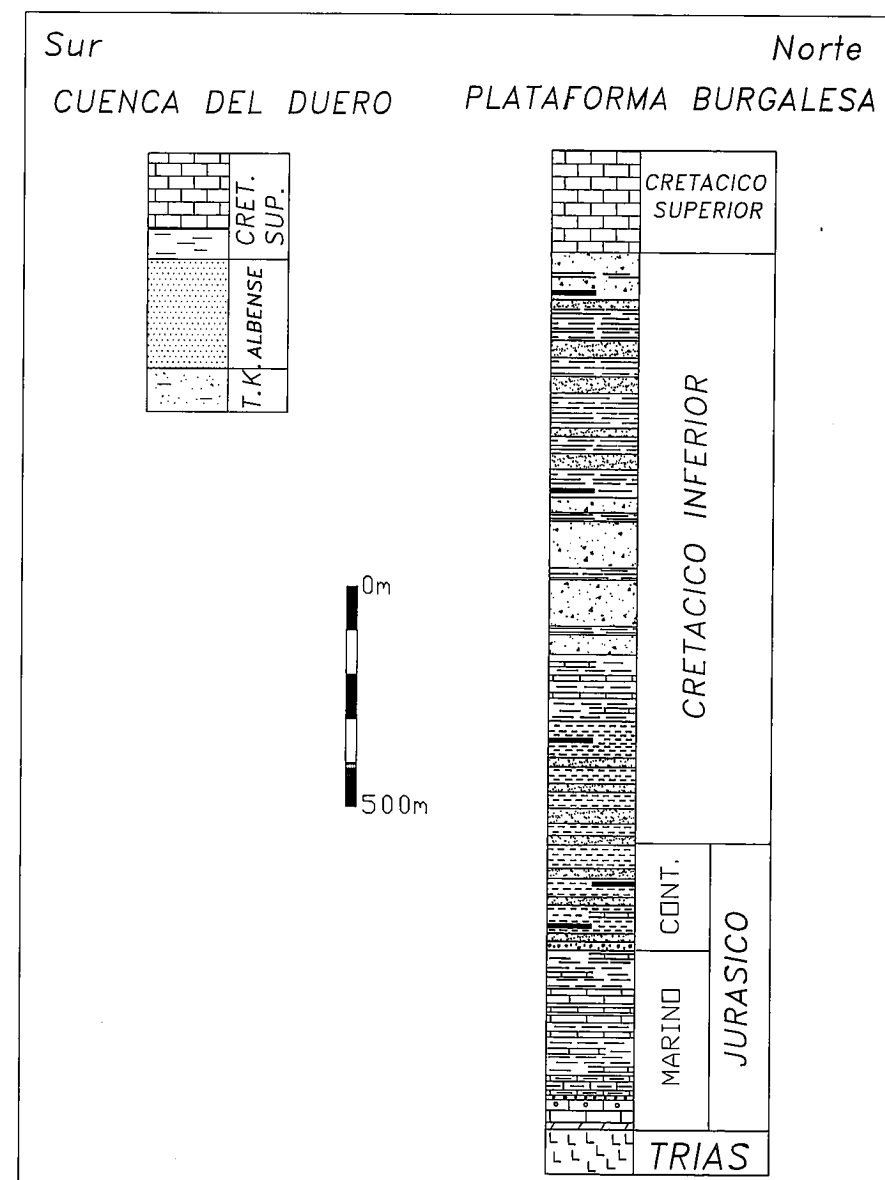
Fig. 2.— Columnas estratigráficas del Mesozoico del NE de la Cuenca del Duero y del SO de la Cuenca Cantábrica
